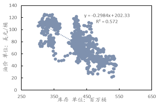
图 25：2010-2026.09 美国商业原油库存与布伦特油价相关性
