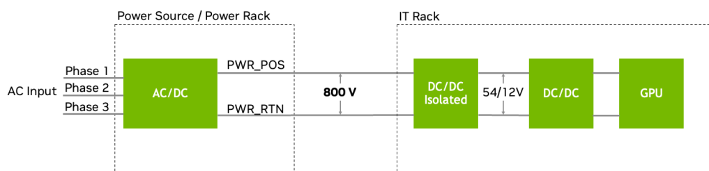
图表15：向 IT 机架分配 800VDC 电源，并将 DC/DC 电源转换为 12V 电源供 GPU 使用
