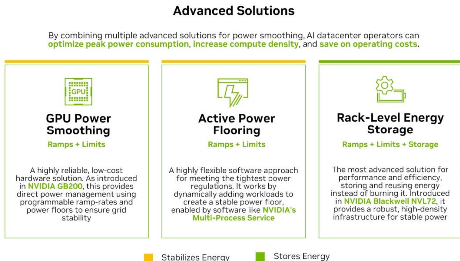
图12: NVIDIA 面向 AI 工厂的多层电源稳压与储能技术
