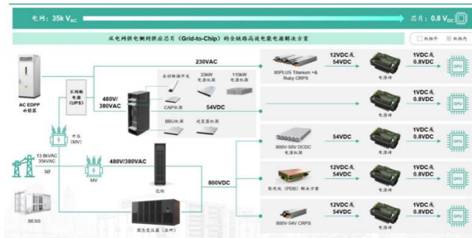
图表18: 麦格米特可提供从电网供电侧到供应芯片的全链路电源解决方案
