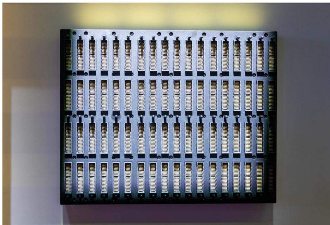
图表3: NVIDIA Kyber Rubin NVL576 采用正交背板实现机柜内全互联
