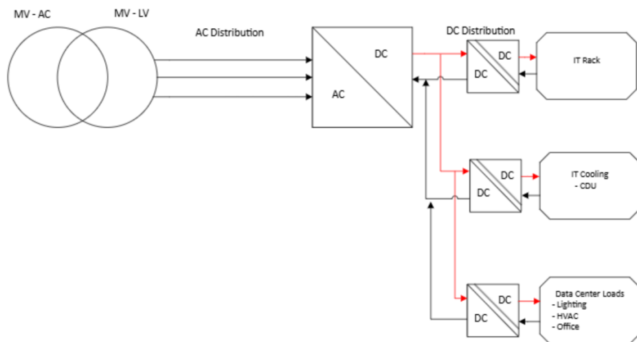
图表16: OCP 白皮书给出的数据中心的完整 LVDC 配电方案
