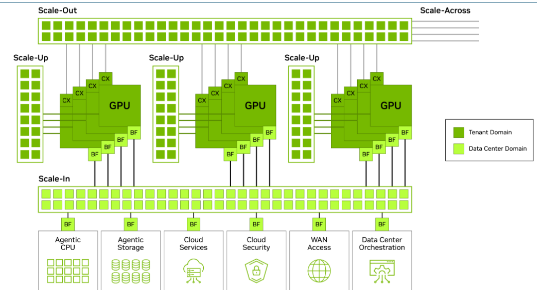
图表20：横向扩展（scale-out）、纵向扩展（scale-up）和跨域扩展（scale-across）增强了计算连接性，而向内扩展则用于连接、保护、配置和监控计算域周围的基础设施。
