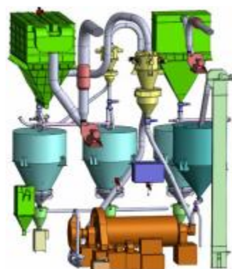
图2：矿物和固废材料粉碎自动化处理产线产品展示
