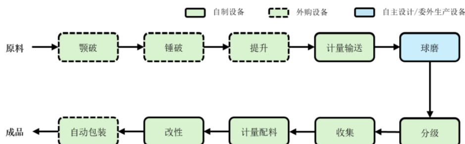
图5: 矿物和固废材料粉碎自动化处理流程与设备
