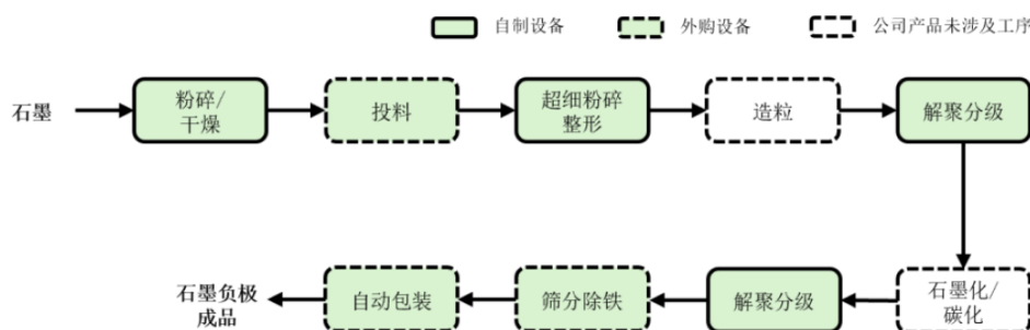
图4: 石墨负极材料生产流程与设备
