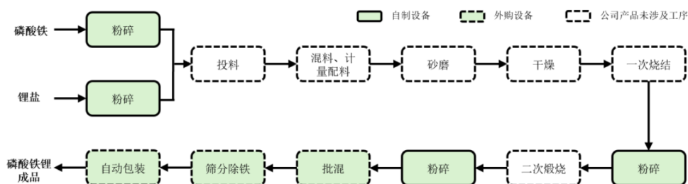
图3：磷酸铁锂正极材料生产流程与设备
