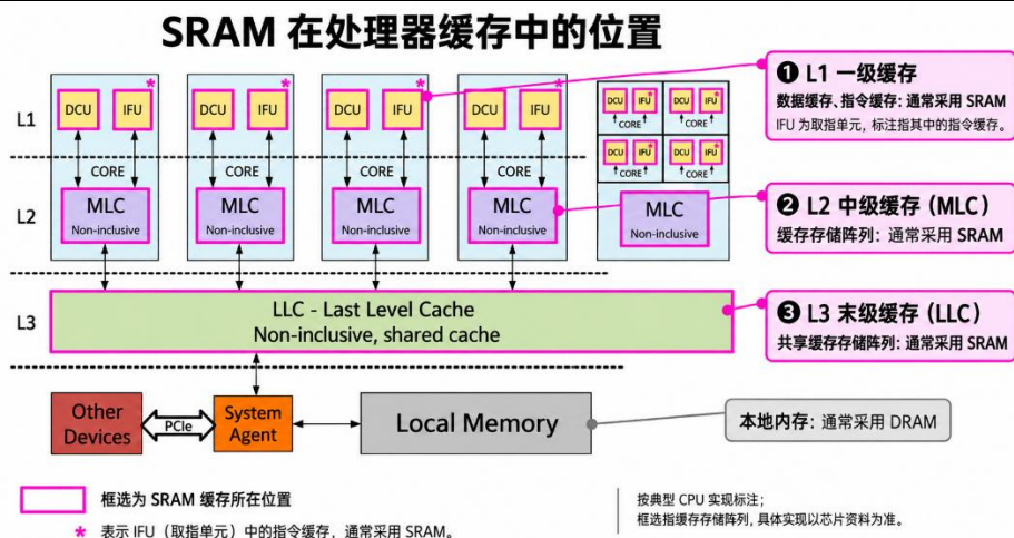
图3：为兼顾速度、容量与成本，CPU 缓存采用分级设计
