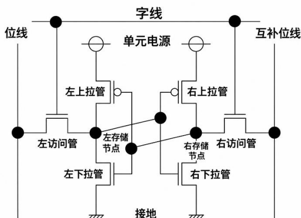
图2：六晶体管（6T）SRAM 存储单元为应用最广泛的 SRAM 位单元架构
