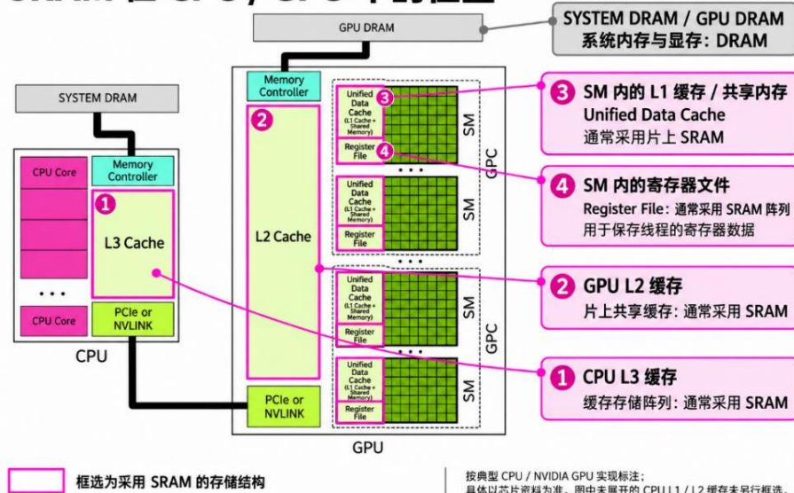
图4：除 CPU 外，GPU 等 AI 芯片也采用 SRAM 阵列来支撑并行计算
