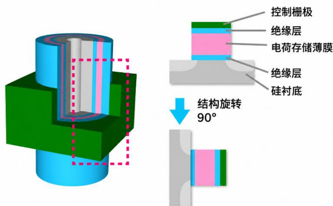
图8：在 BiCS FLASH（铠侠自研 3D NAND FLASH）存储单元中，电子在穿过柱体中心的电极（图中灰色部分所示）和电荷存储膜（粉色部分）之间进行交换
