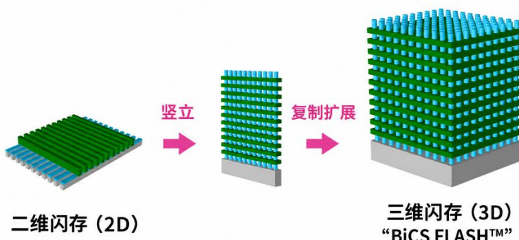
图9：2D NAND 存容量扩展受限，3D NAND 依靠垂直堆叠扩容，已成为主流技术
