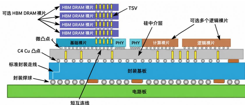
图7：HBM以硅通孔将多层DRAM裸片垂直堆叠，经硅中介层与GPU并排封装
