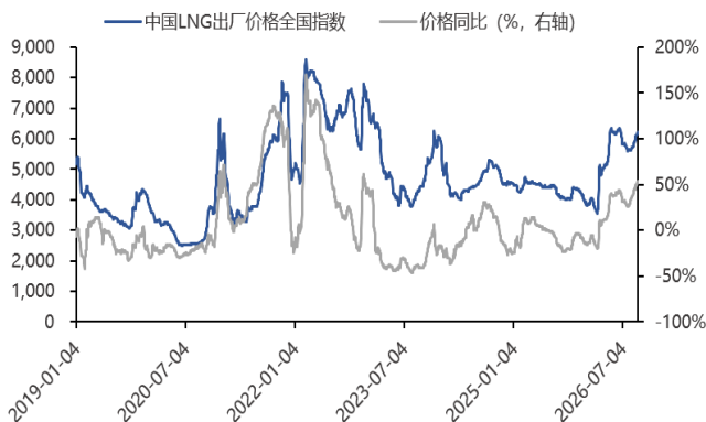
图表35: 中国LNG出厂价格走势 (元/吨)
