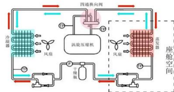
图10: 新能源汽车热泵空调热管理的工作原理
