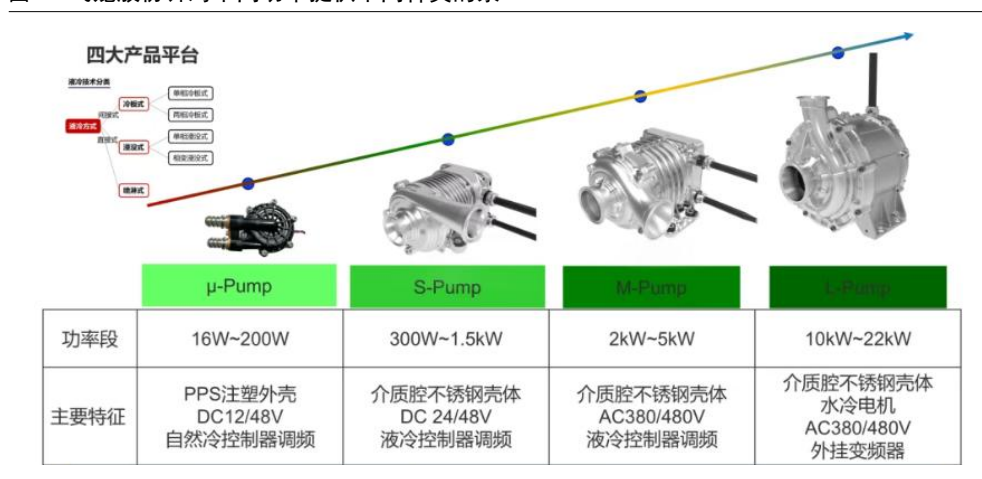
图25: 飞龙股份针对不同功率提供不同种类的泵
