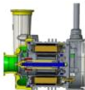
图24: 电子水泵的主要结构
