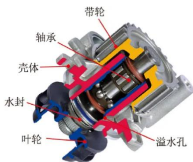
图23: 传统机械水泵的主要结构
