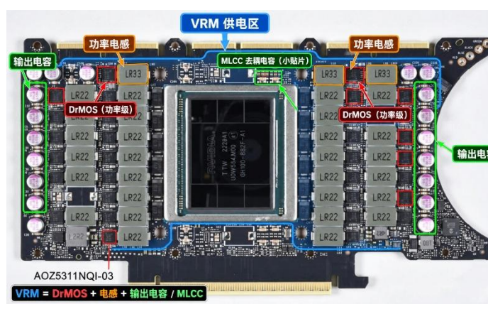
图23: H100 VRM 供电区展示
