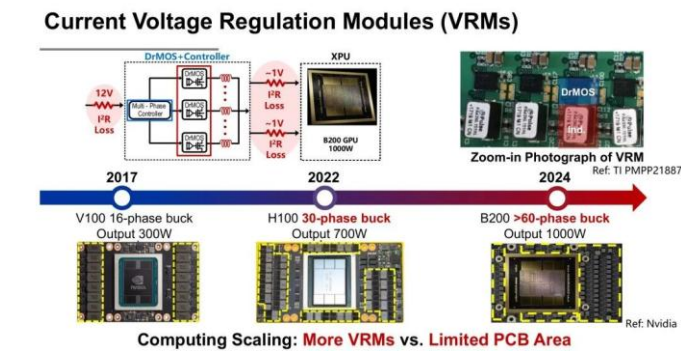
图25: VRM 相数的指数级膨胀
