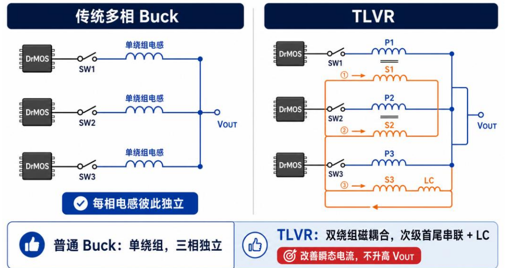
图29： TLVR 通过次级绕组及补偿电感构建耦合回路
