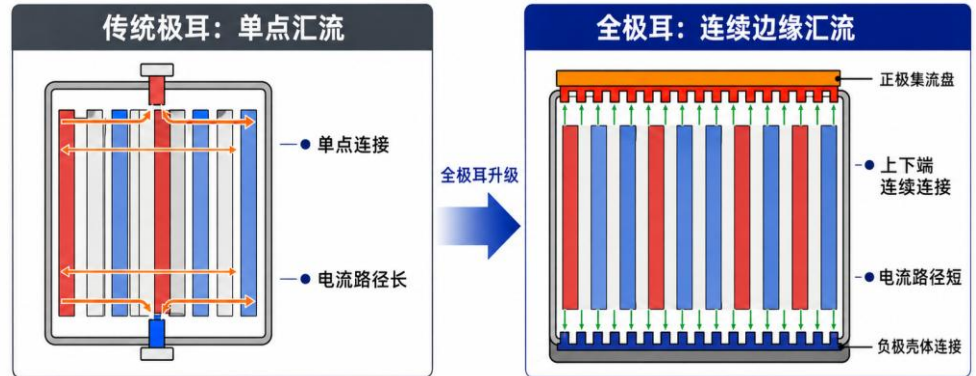
图12：全极耳结构具备低内阻、低温升、高倍率等优势
