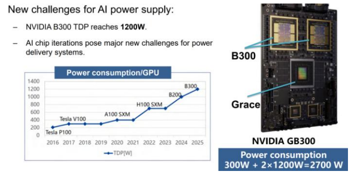
图26: GPU 功率持续提升
