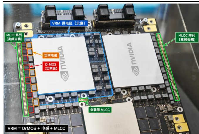
图24: GB200 VRM 供电区展示
