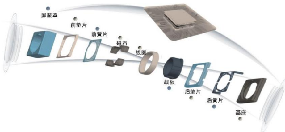
图15: 摄像头马达驱动芯片的组装结构
