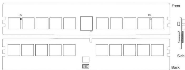
图9: JEDEC 关于 RDIMM 类型 DDR5 内存模组的标准图示
