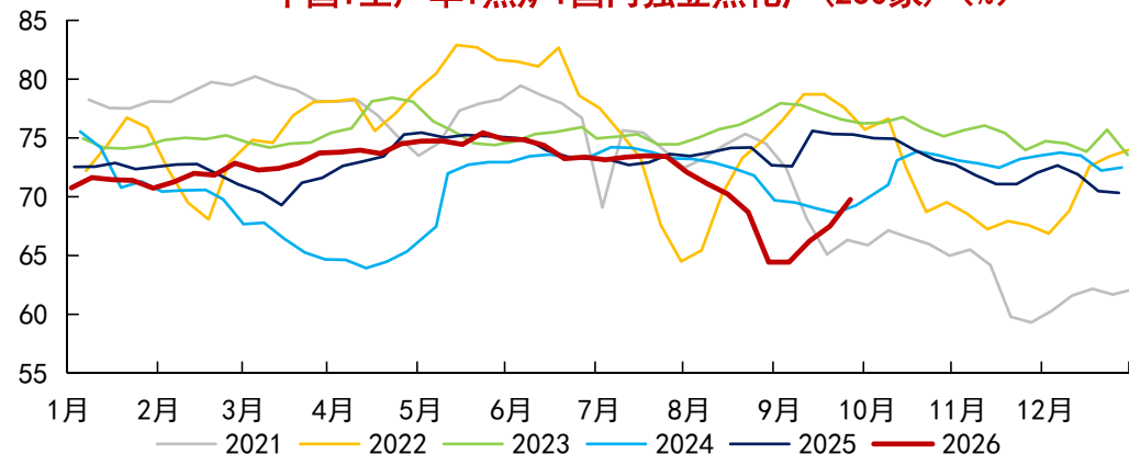
中国:生产率:焦炉:国内独立焦化厂(230家)(%)
