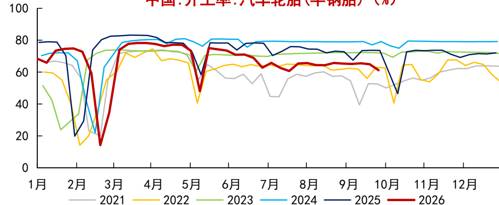
中国:开工率:汽车轮胎(半钢胎)(%)
