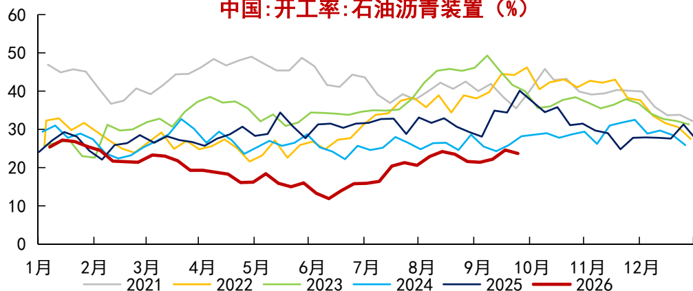
中国:开工率:石油沥青装置 (%)
