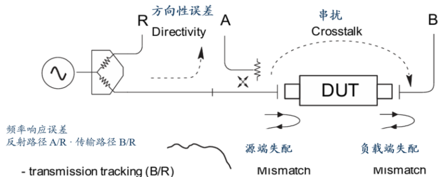
图：VNA测量误差分布——信号泄漏、端口失配及频响偏差共同影响结果
