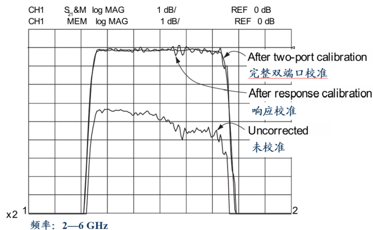
同一滤波器的传输特性 S21
