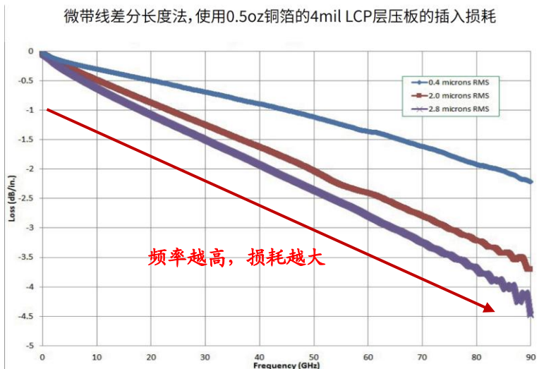
图：高频化放大PCB传输损耗
