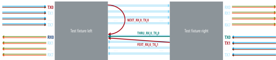
图：PCIe x8 电缆合规性测试
