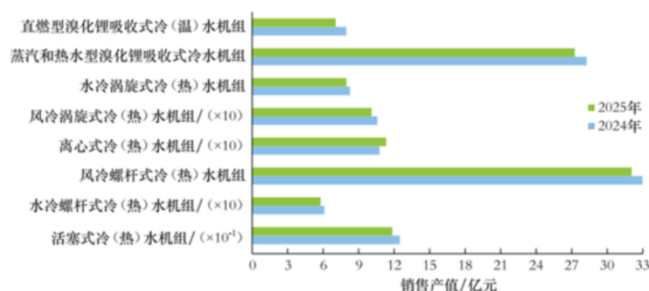
图 19：2024—2025 年各类（热）水机组销售产值对比
