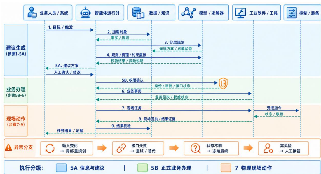
图 11 任务规划、专业求解与受控执行时序
