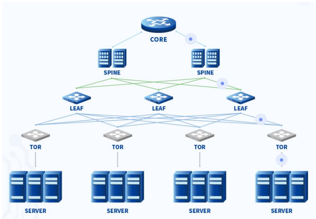
图8：数据通信类产品应用拓扑图
