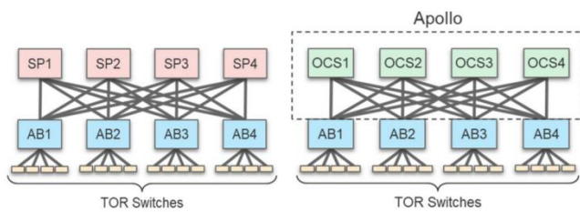
图30: Apollo OCS 架构相比传统网络架构有着更低的功耗和成本
