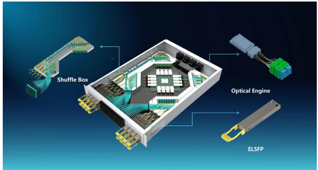
图25: CPO 以及三大核心组件图示
