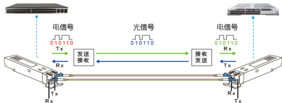
图15: 光模块工作原理图
