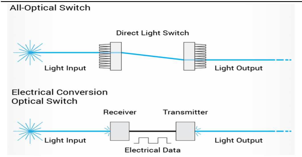
图29：OCS 与电交换机的差异在于能够直接进行光信号交换
