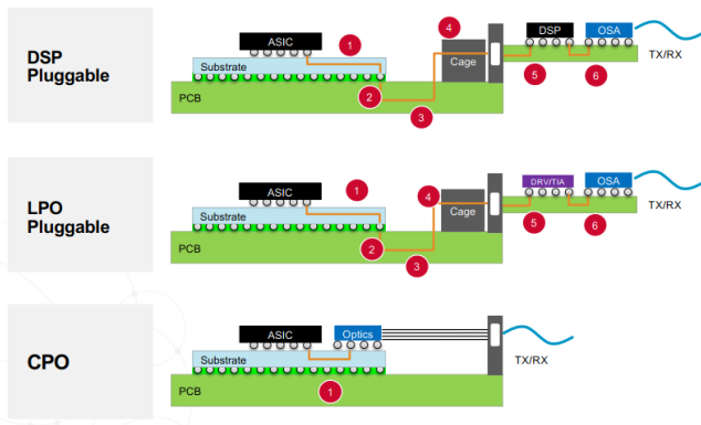
图22: CPO 技术将光引擎与交换芯片封装在同一基底
