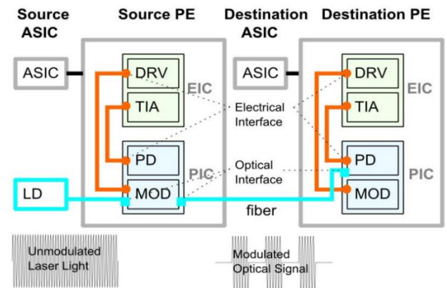
图23: CPO 技术中光引擎是完成光电转换的核心部分
