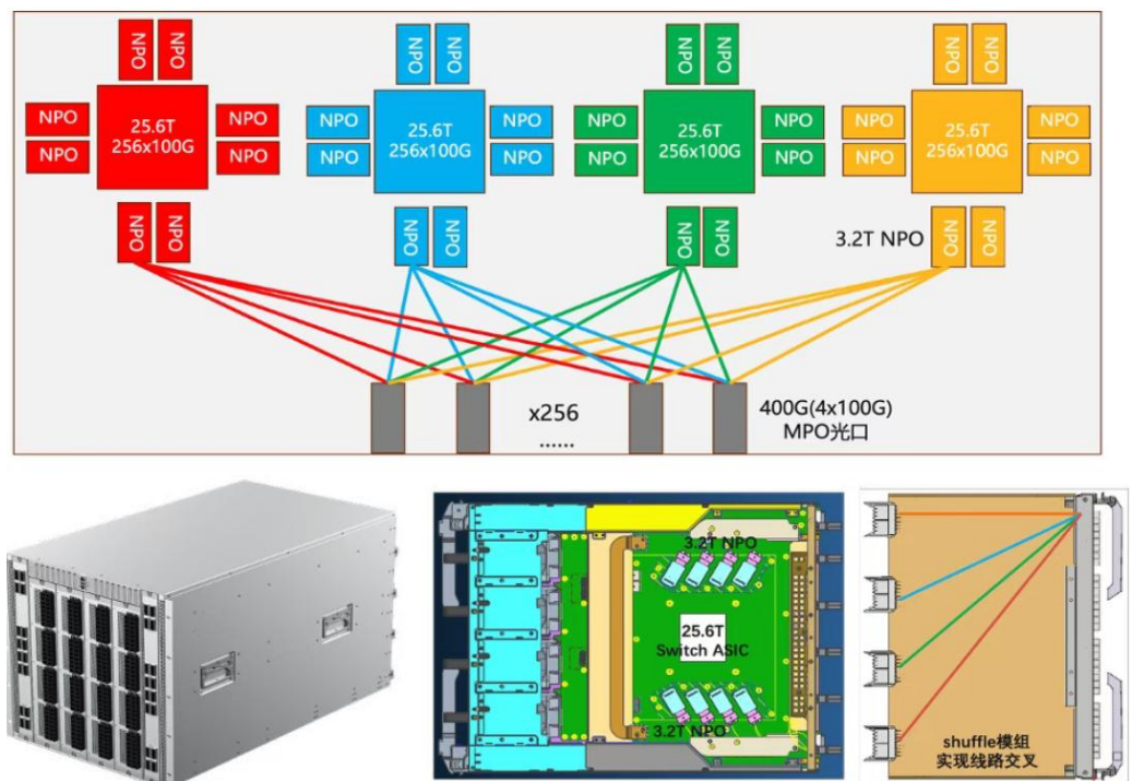
图27：阿里云将 3.2T NPO 技术应用于新一代四芯片交换机
