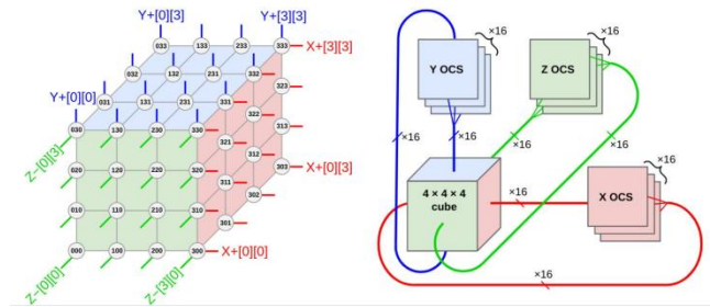
图31: TPU 通过 OCS 连接，组成 3D Torus 拓扑
