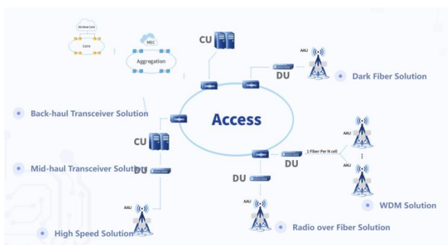
图6: 无线接入类产品应用拓扑图
