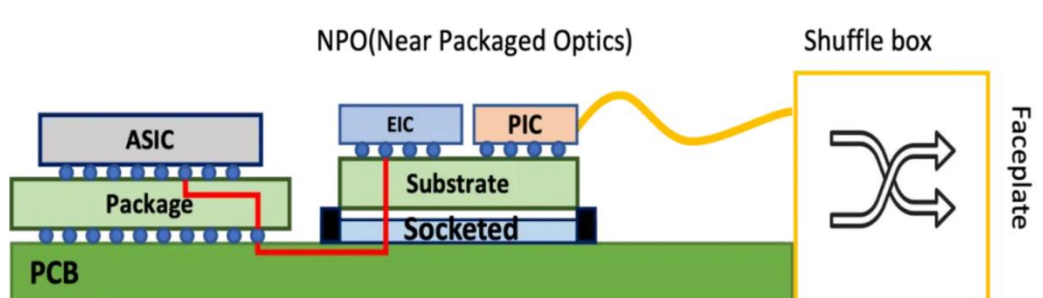
图26: NPO 技术通过插槽实现光引擎的可插拔连接
