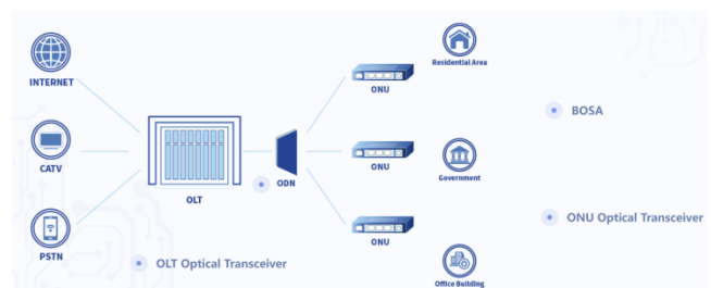
图7: 固网接入类产品应用拓扑图
