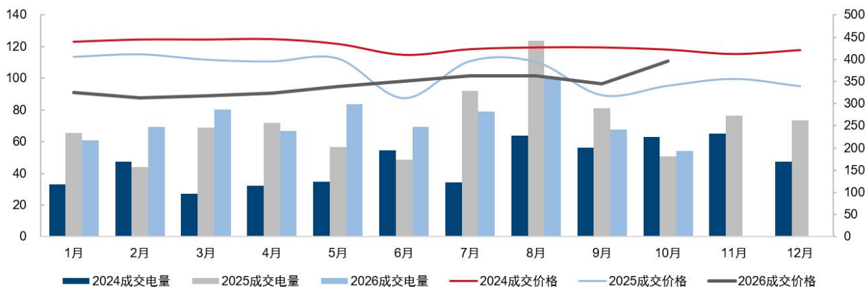
图1：2024 年、2025 年及 2026 年 1-10 月江苏电力集中竞价交易结果
