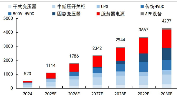
图 30: 全球各类 AIDC 电力设备市场空间测算 (亿元)
