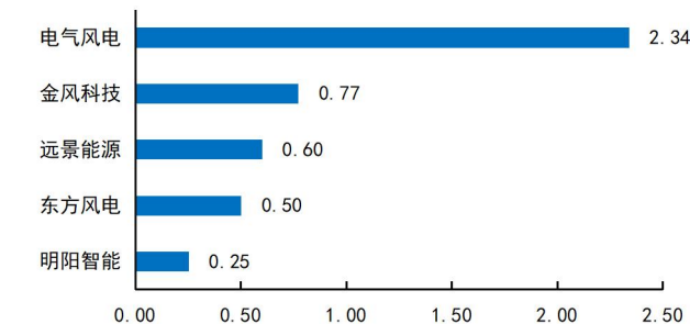
图10：2026年1-9月风电整机制造商中标情况统计（GW）（国内海上项目）
