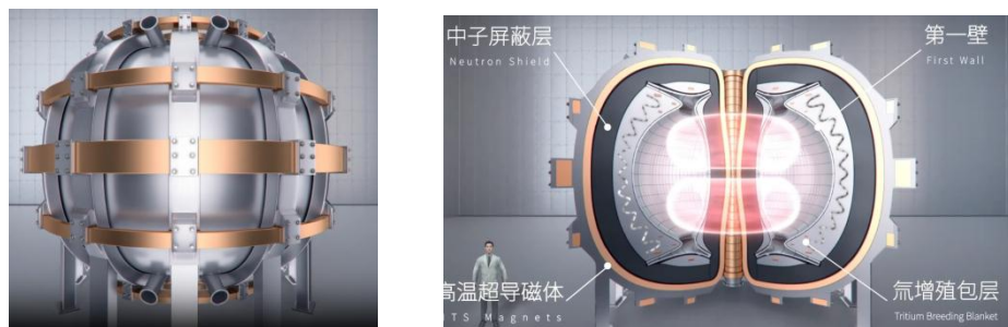
图 27：星环聚能球形托卡马克示意图
