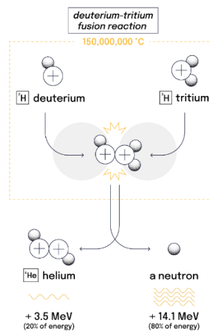
图 2：实验室的氘氚聚变反应
