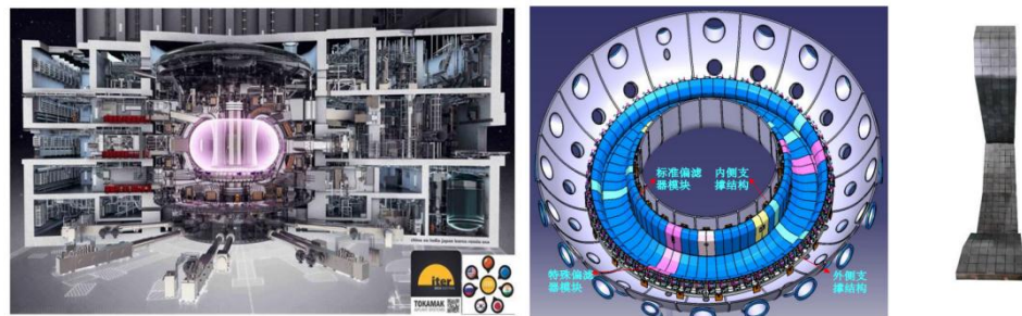
图 20：国光电气 ITER 主体托卡马克装置和偏滤器示意图
