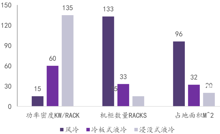
图表21：液冷同比风冷散热能力（2MW 机房）
