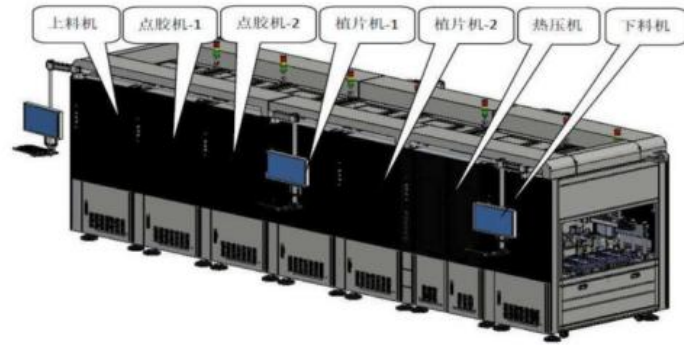
图5: 公司生产的全自动芯片植散热片机
