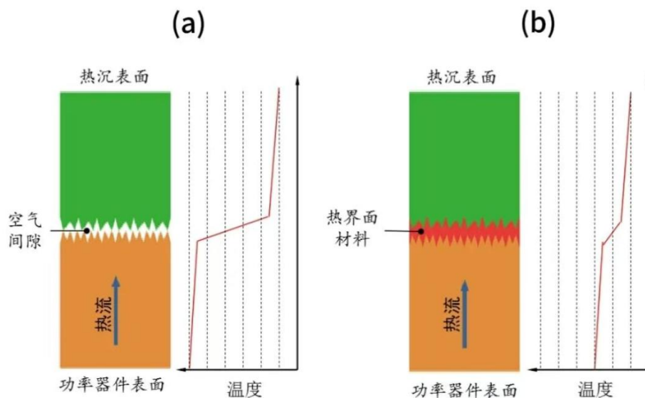
图7：热界面材料的工作原理示意
