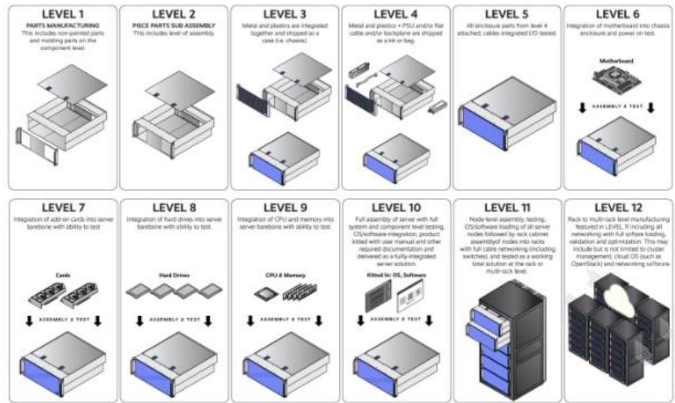
图26：服务器机柜组装，主要分为 12 个阶段
