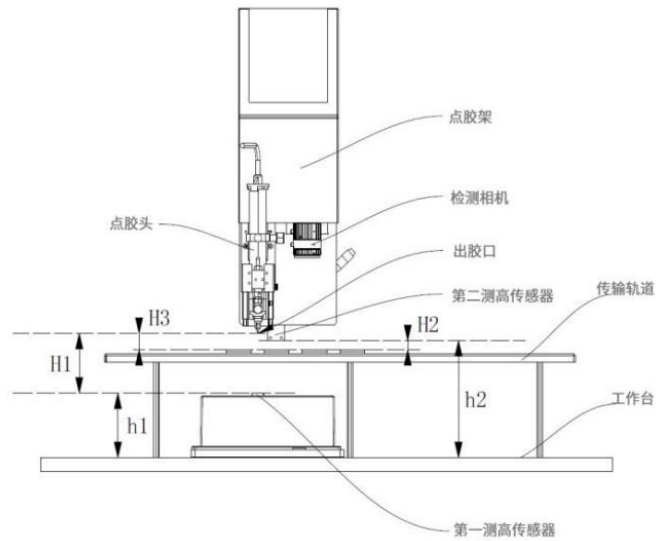
图6: 在芯片植盖工艺中，点胶设备是属于核心自动化设备
