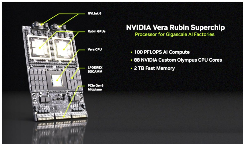
图11: SOCAMM 在英伟达 Vera Rubin 主板的应用
