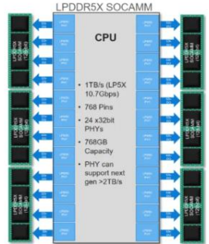
图10: POP 焊接形式维修困难，SOCAMM 可插拔是出路
