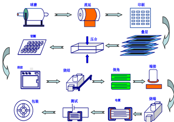
图11: MLCC 生产工艺
