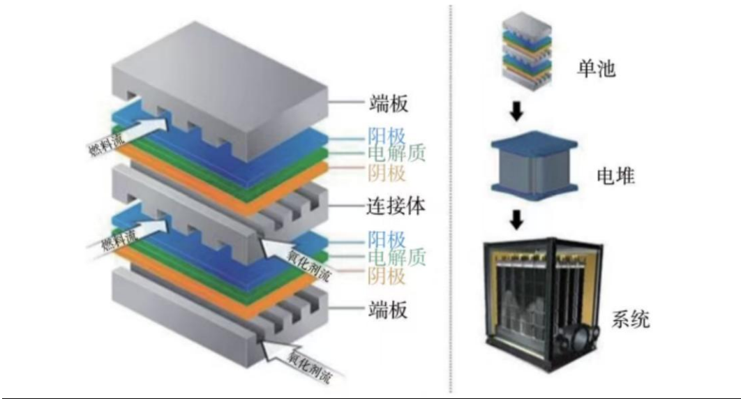
图16: SOFC 发电单元和系统集成图
