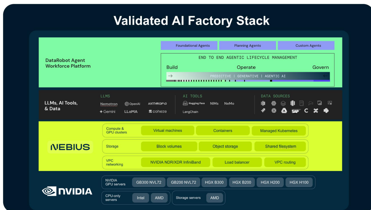
图 15: Nebius AI Token Factory 架构
