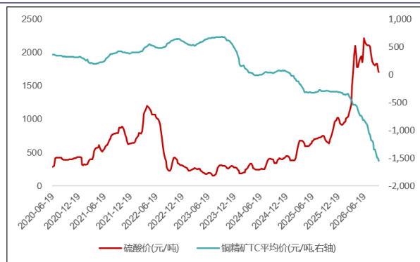
图表6：2026 年 7 月初硫酸见顶，TC 价格继续下跌
