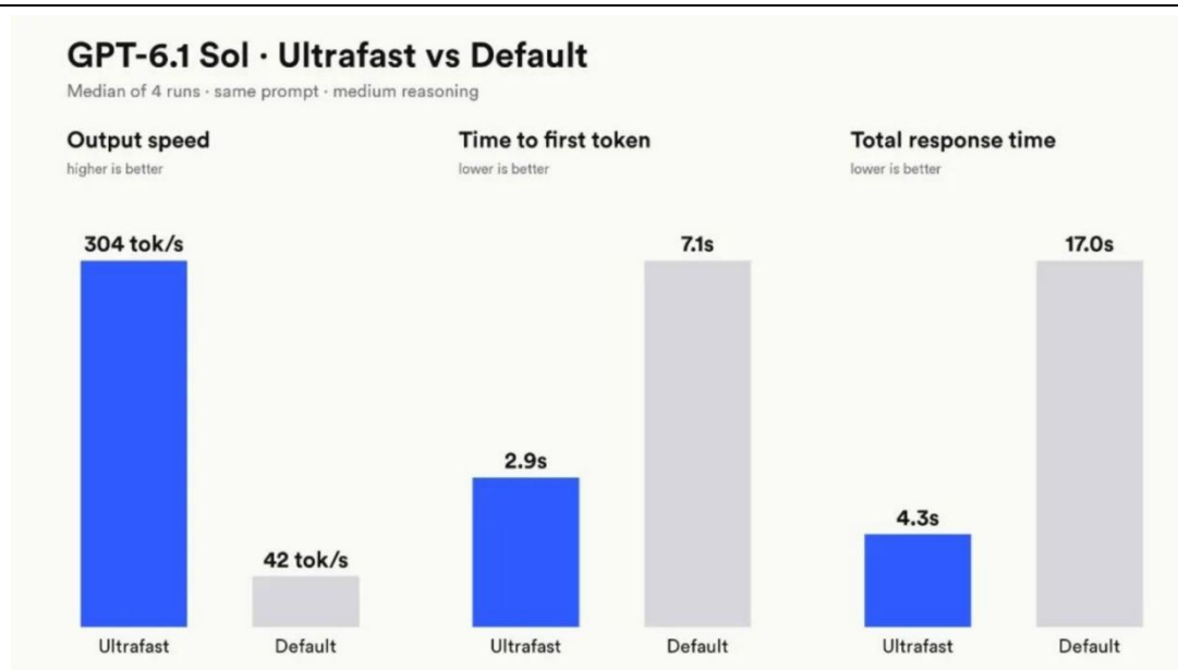
图表 7：GPT-6.1 Sol 极速版与标准版输出性能与响应延迟实测对比
