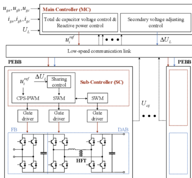
图：SST分为两级控制架构
