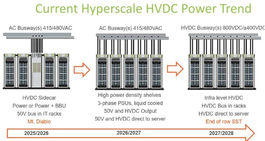
图：AIDC高压直流供电由侧柜方案向设施级SST演进
