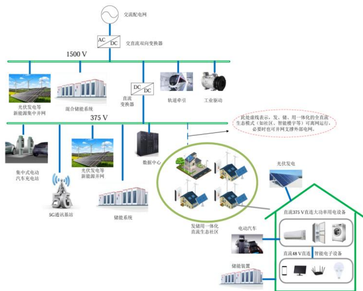
图：低压直流配电系统架构示意图
