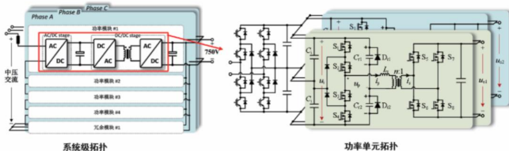
图：典型SST系统拓扑图
