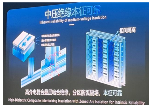
图：四方股份数智1.0 SST模块绝缘设计
