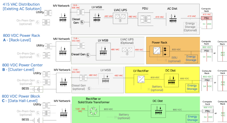
图：从415伏交流（上方）到800伏直流配电（下方）的转变
