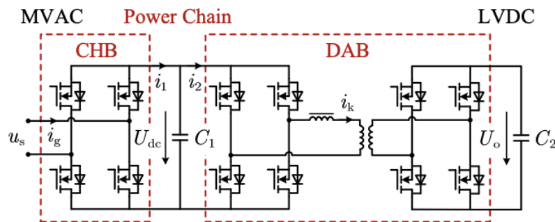
图：SST框架拓扑图
