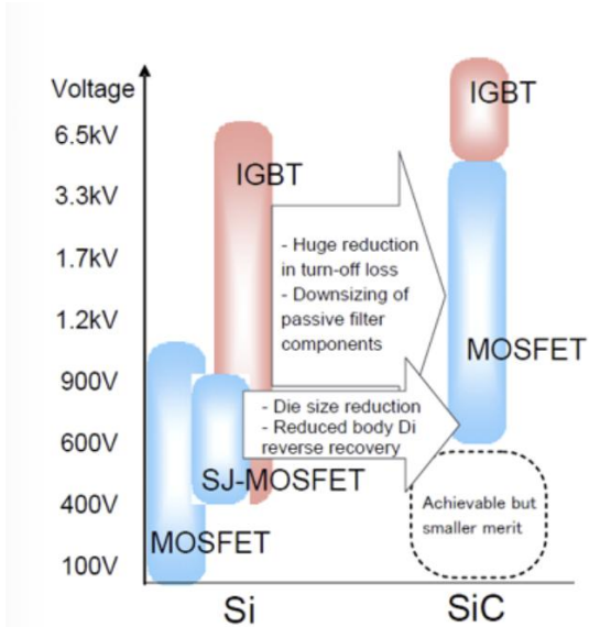
图：SiC MOSFET更适配于SST整流
