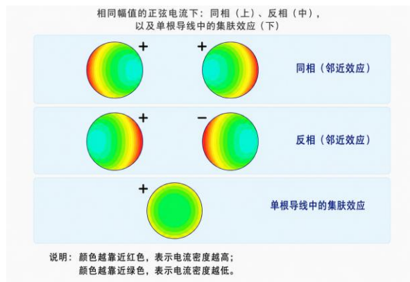
图：趋肤、邻近效应示意图
