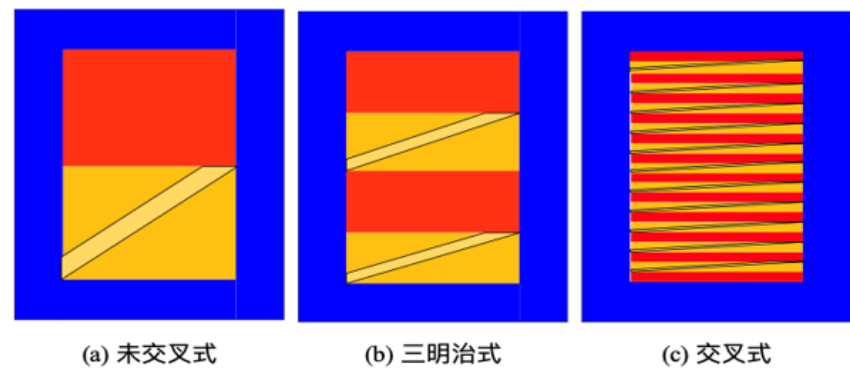
图：三种绕组排布方式
