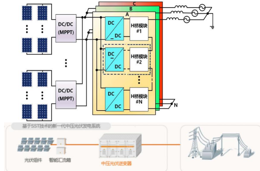
图：阳光电源基于SST技术的6MW/35kV中压直挂光伏并网逆变器系统
