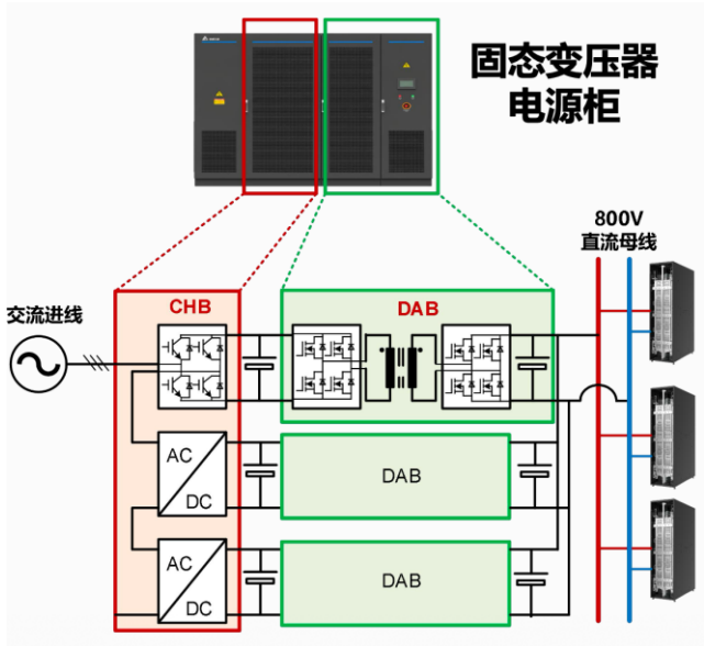
图：SST整体架构图
