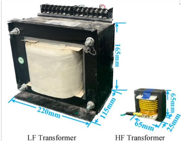
图：高频变压器与体积明显优于传统工频变压器
