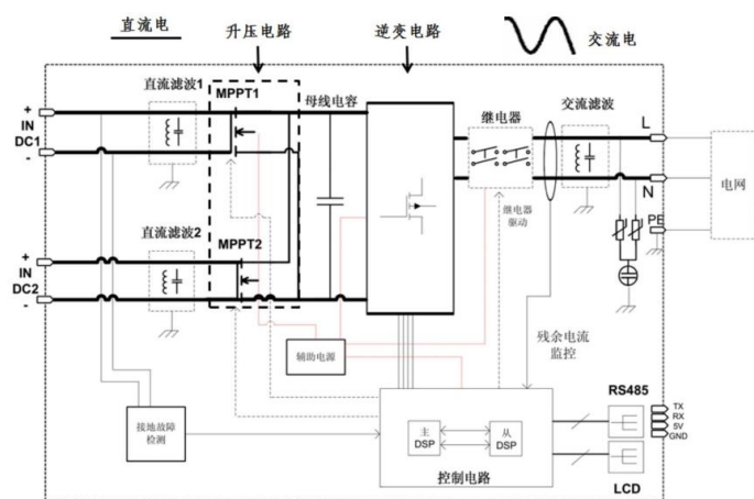
图：典型光伏逆变器系统拓扑图
