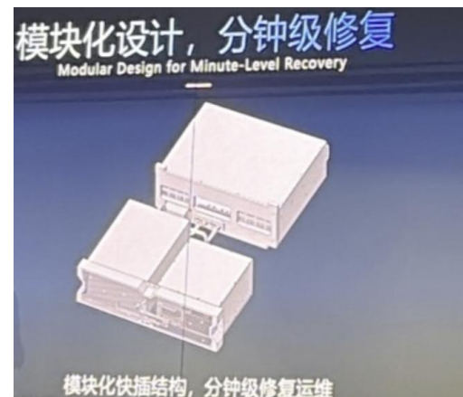
图：四方股份数智1.0 SST模块化设计
