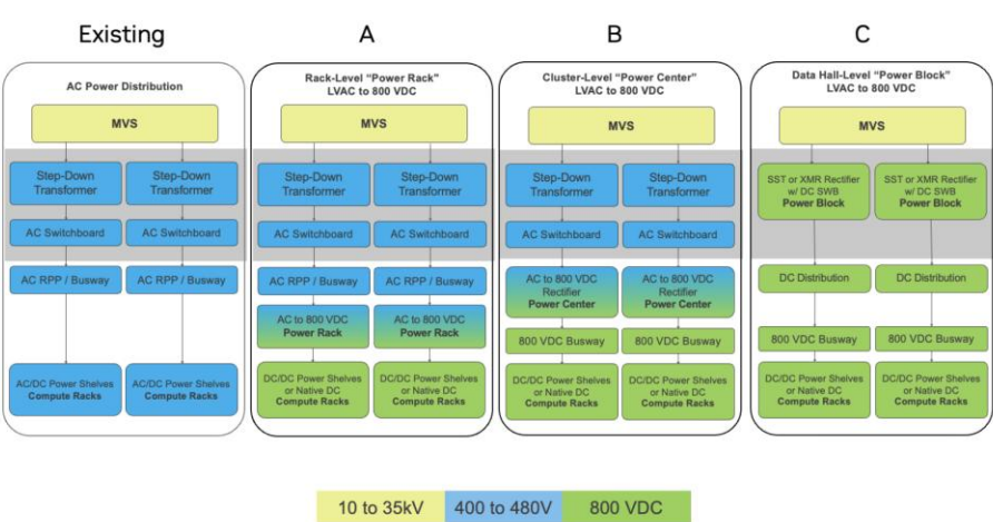
图：英伟达白皮书2.0中阶段C将采用SST作为800V DC架构的终极方案
