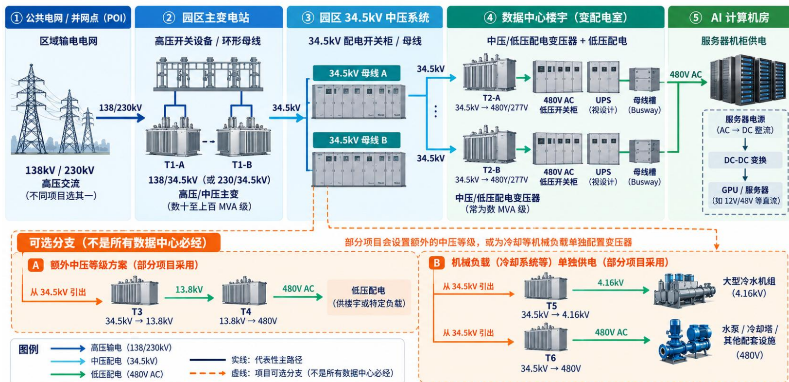
图：美国超大型AI算力中心配电架构-34.5kV是中压的标准方案
