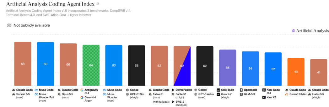
图 5：大模型编程能力排名
