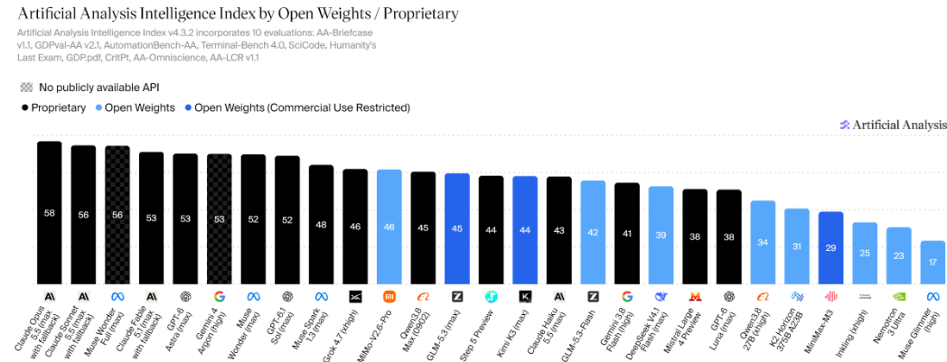
图 3：开源及闭源模型能力对比及智能能力指数
