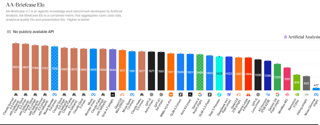
图 4：大模型智能体工作任务能力对比
