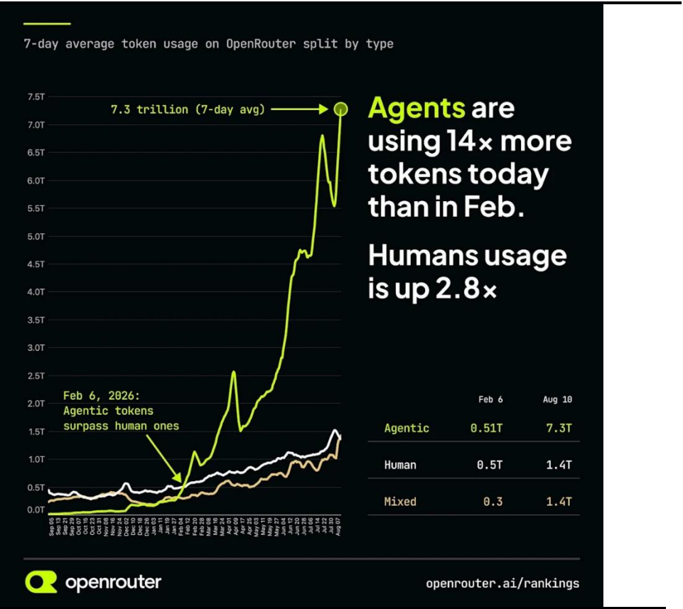
图 8：2 月 6 日至 8 月 10 日，agents 7 天平均 token 使用量上涨 14 倍，而人类使用量上涨 2.8 倍
