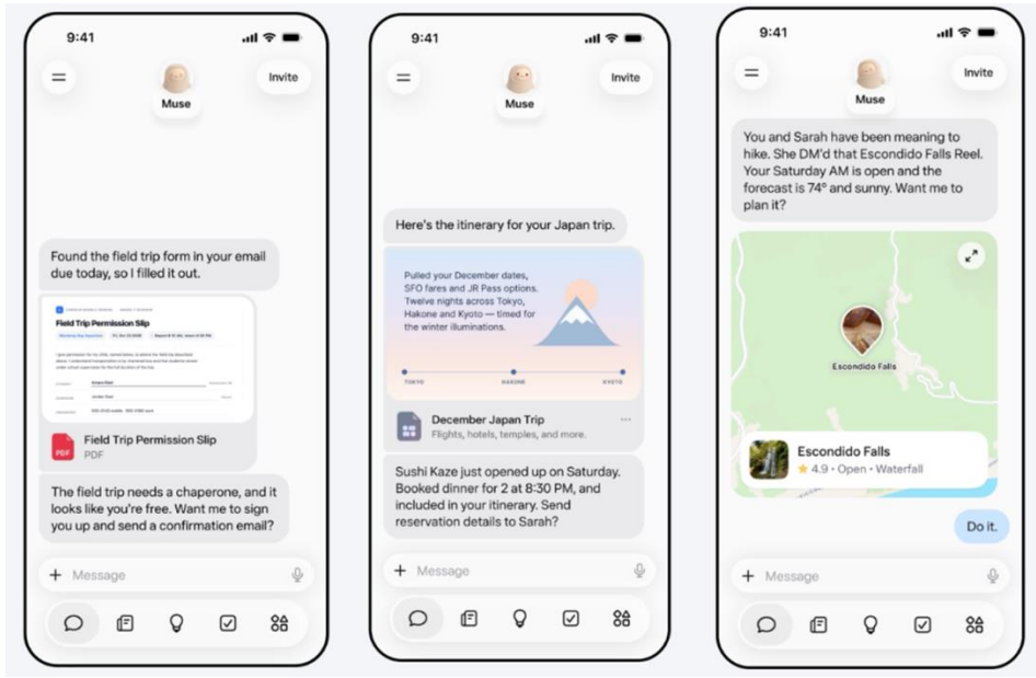
图 22: Meta Muse
