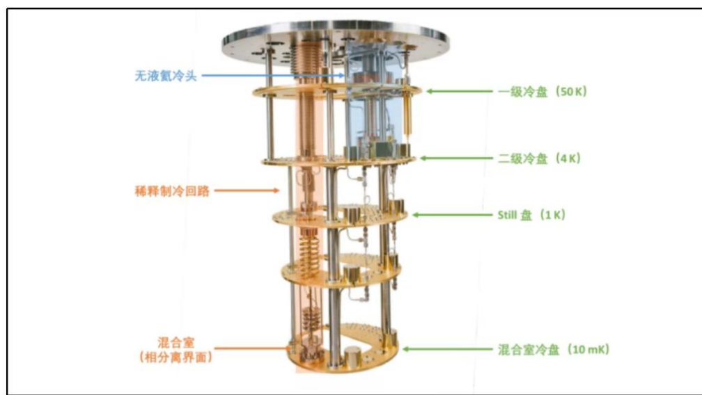
图1：稀释制冷系统呈“金字塔”型结构
