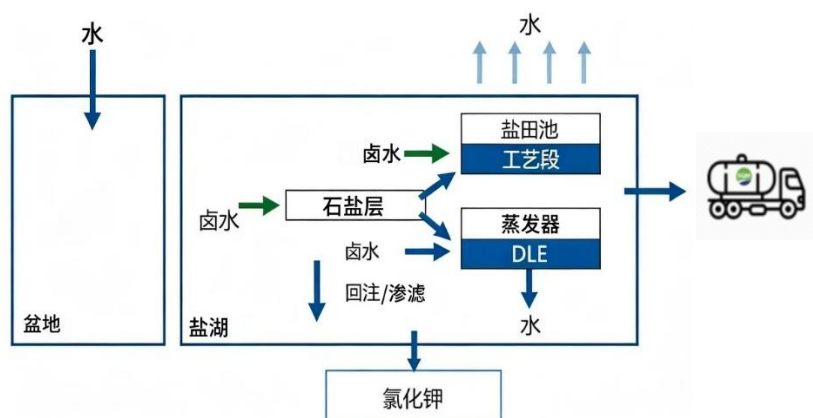
图表 37: Salar Futuro 项目整体工艺框图
