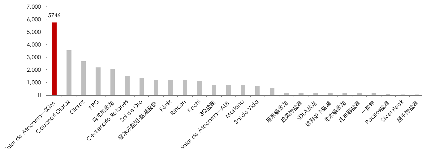
图表 2：全球主要盐湖资源量排名（万吨 LCE）
