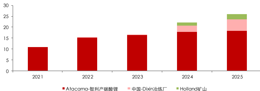
图表 34：2020-2025 年锂资源产量（折 LCE，万吨）
