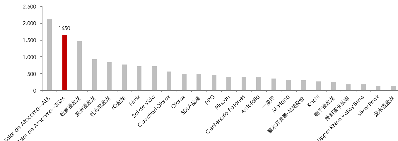
图表 3：全球主要盐湖 Li 离子浓度（ppm）
