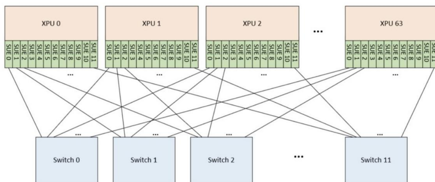
图17: XPU 通过部署 12 个 SUE 并使用 12 台 64 个端口的以太网交换机实现全交换连接（示例）
