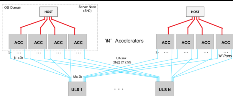
图20: 基于 UALink 的多加速器系统
