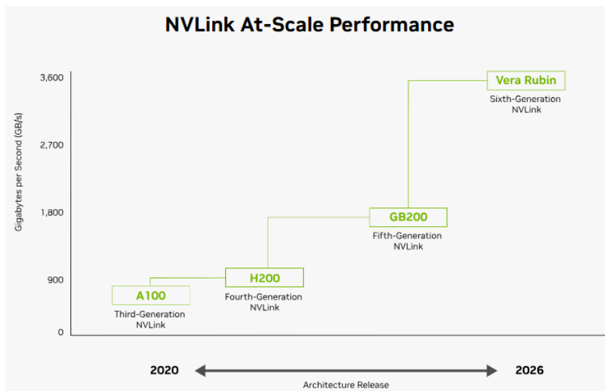
图10: NVIDIA 核心 GPUxNVLink 架构演变史
