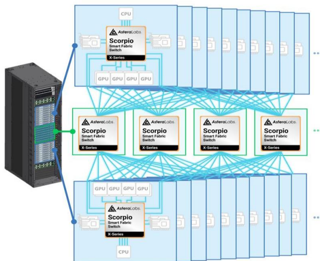
图7: 利用 Scorpio X-Series 320 Lane 实现的 High Radix, Multi-level Switch Scale-up 组网
