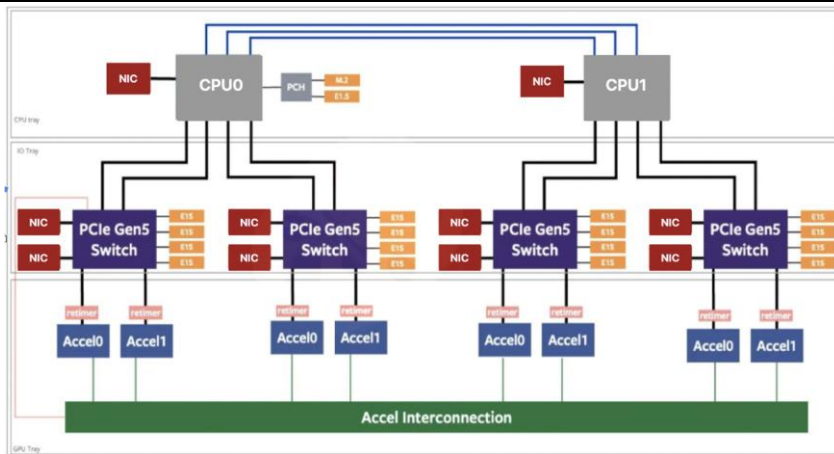
图3：PCIe 是 AI 服务器柜内 CPU-外设最核心的互连总线
