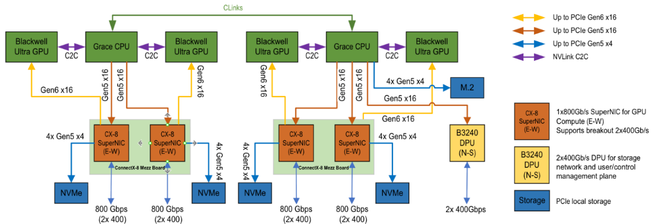
图5: PCIe 同 NVLink C2C 一起承担 NVL72 中的 CPU-外设互连
