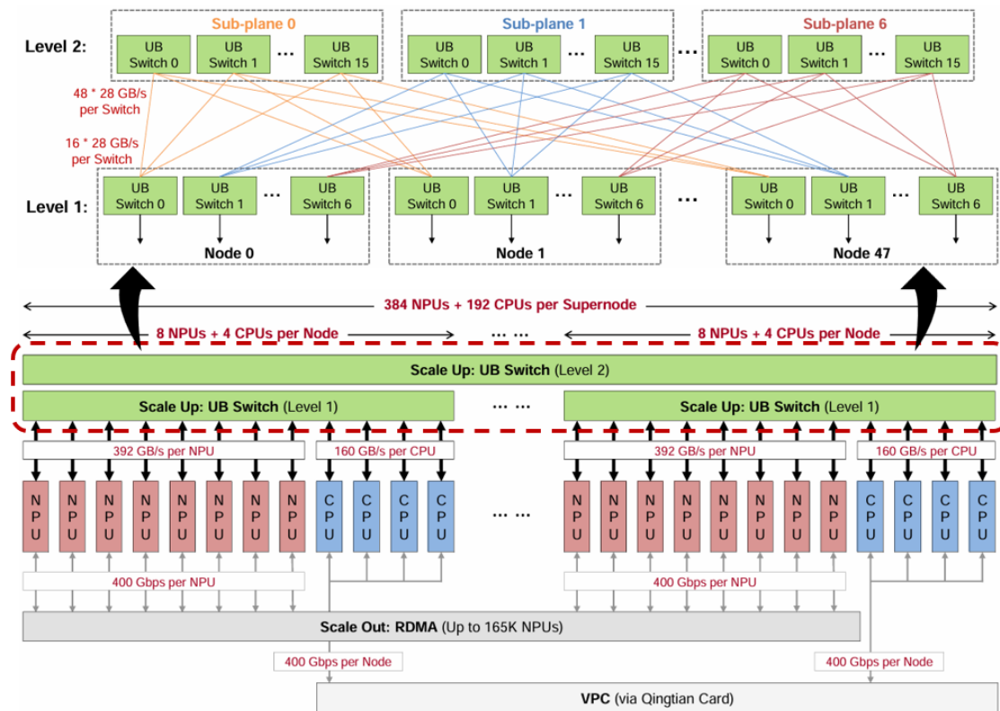
图13: CloudMatrix384 超节点的对等直连硬件架构及 UB 交换系统示意图
