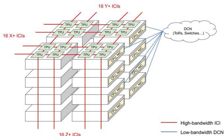
图15: 谷歌 TPUv4 中 TPU 通过 ICI 沿着 x/y/z 三个维度完成互连形成 4x4x4 结构
