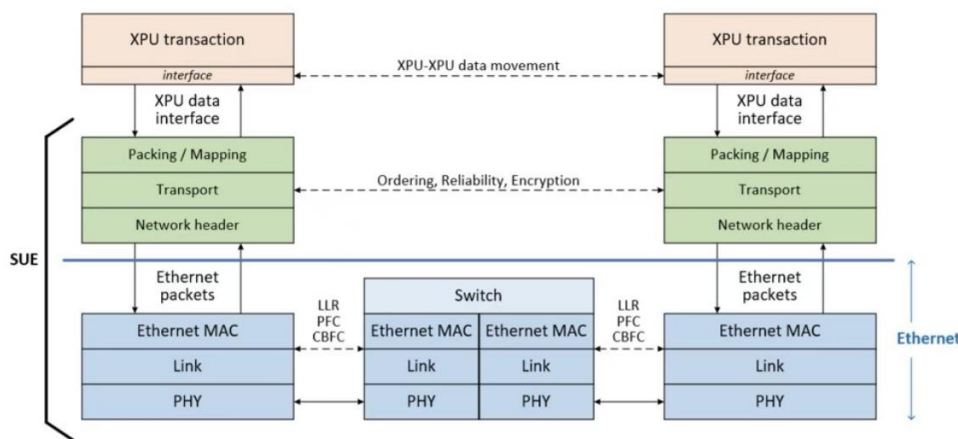
图 16：标准 SUE 协议栈及工作流程示意图
