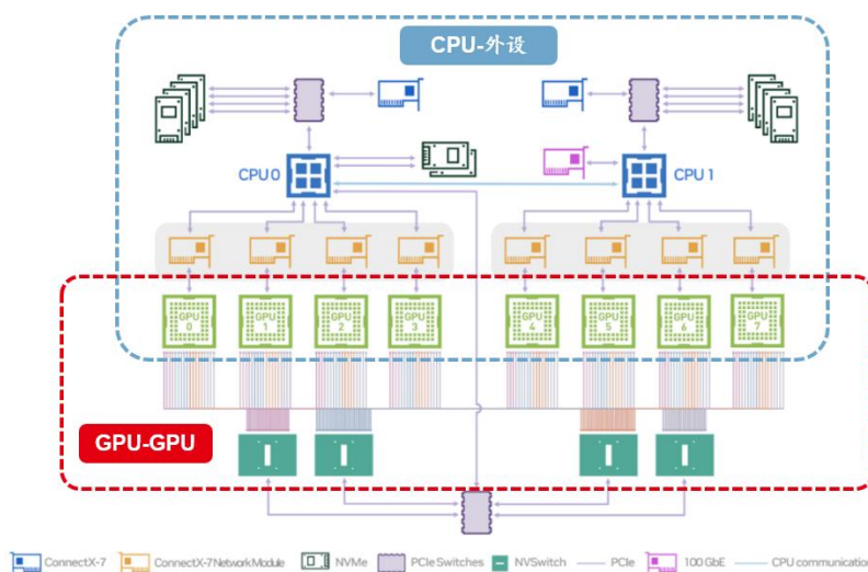
图2：（超）节点（柜）内互连模式可分为“CPU-外设”与“GPU-GPU”
