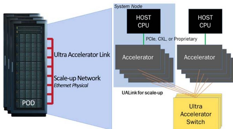
图19: 基于 UALink 的 Scale-Up 机柜架构中的多节点与多平面交换
