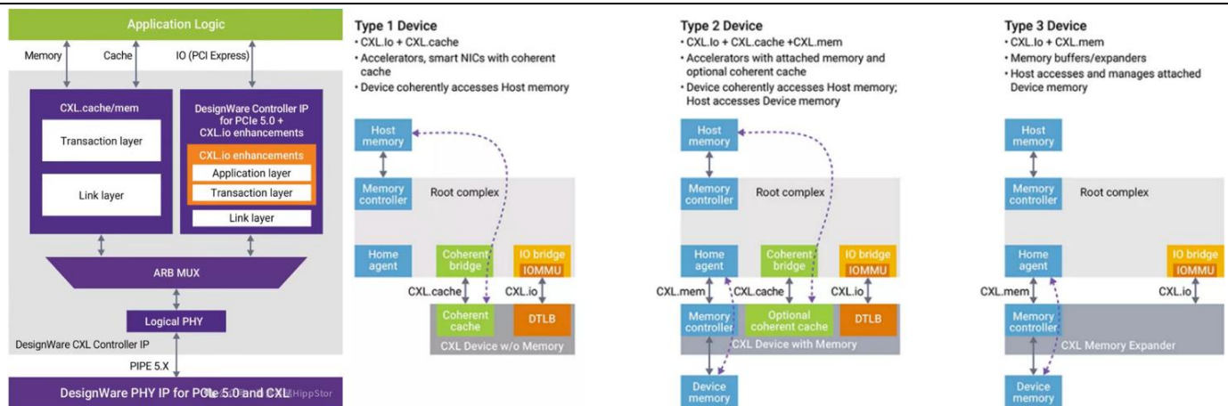
图6: CXL 定义的三类设备及其 PHY、控制器与应用层
