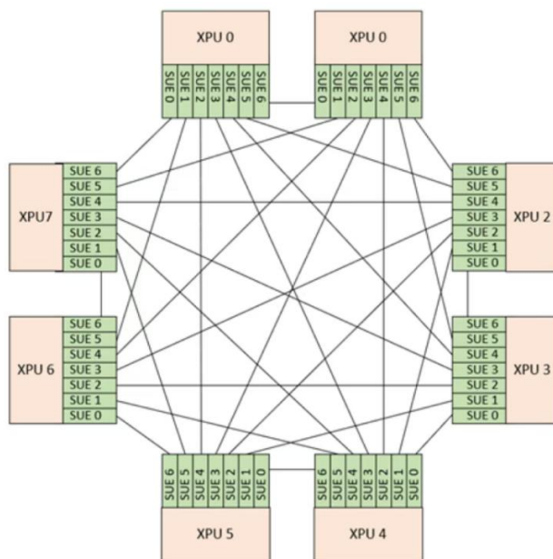
图18: XPU 利用 SUE 直接互连网状拓扑结构（示例）
