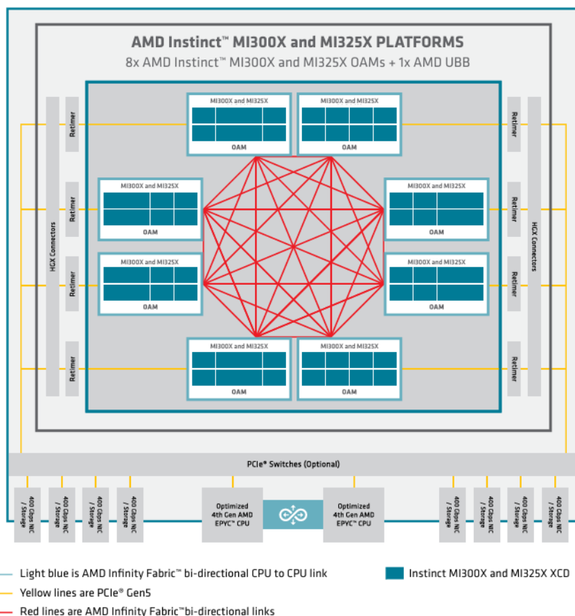
图11: AMD Instinct MI300X&MI325X 平台利用 Infinity Fabric 实现 8GPU 全互连
