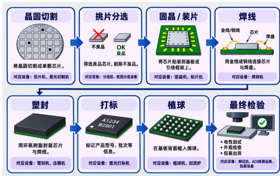
图表 12：传统封装主要工序环节及对应代表性设备
