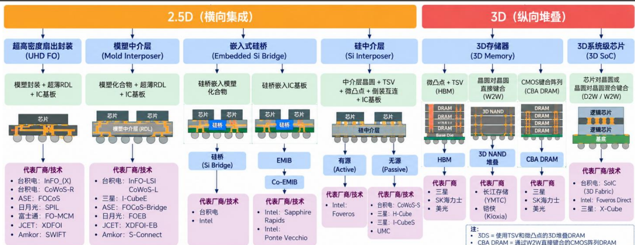
图表 8：2.5D 和 3D 封装基础结构图及代表厂商
