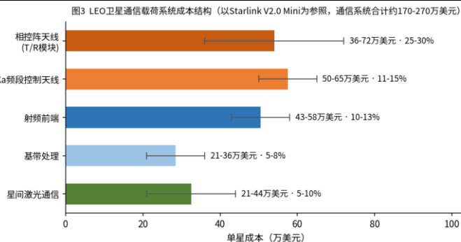
图13 Starlink 通信载荷成本拆分
