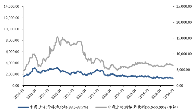
图45：氧化镨、氧化铽价格走势（元/千克）
