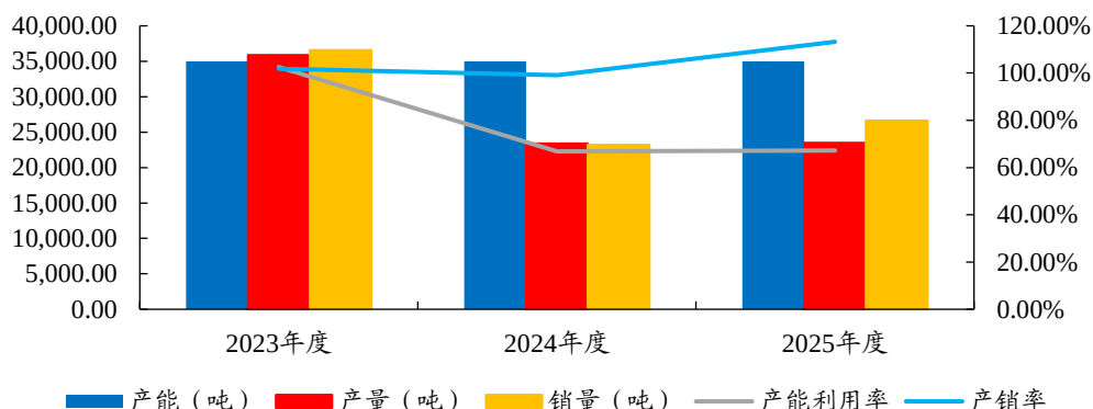
图8：2025 年度，桥梁钢结构产品产能利用率为 67.16%，产销率为 113.25%
