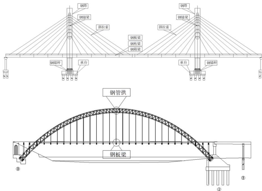
图4：公司桥梁钢结构产品
