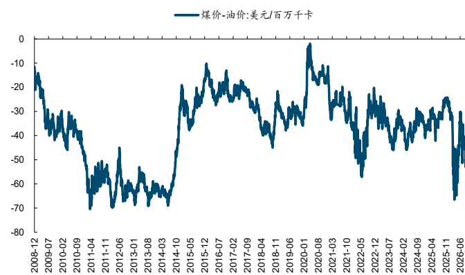
图表19: 目前煤油价差已处于低位
