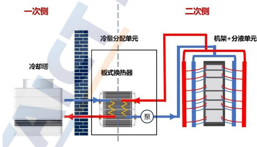
图1：冷板式液冷系统原理图
