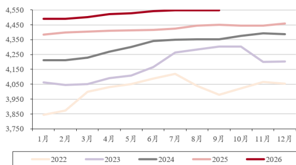
图表31. 中国电解铝在产产能（万吨）
