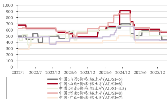
图表39. 四省铝土矿价格 (元/吨)
