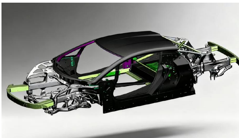
图 9：仰望 U9Xtreme (U9X) 车身 3D 打印
