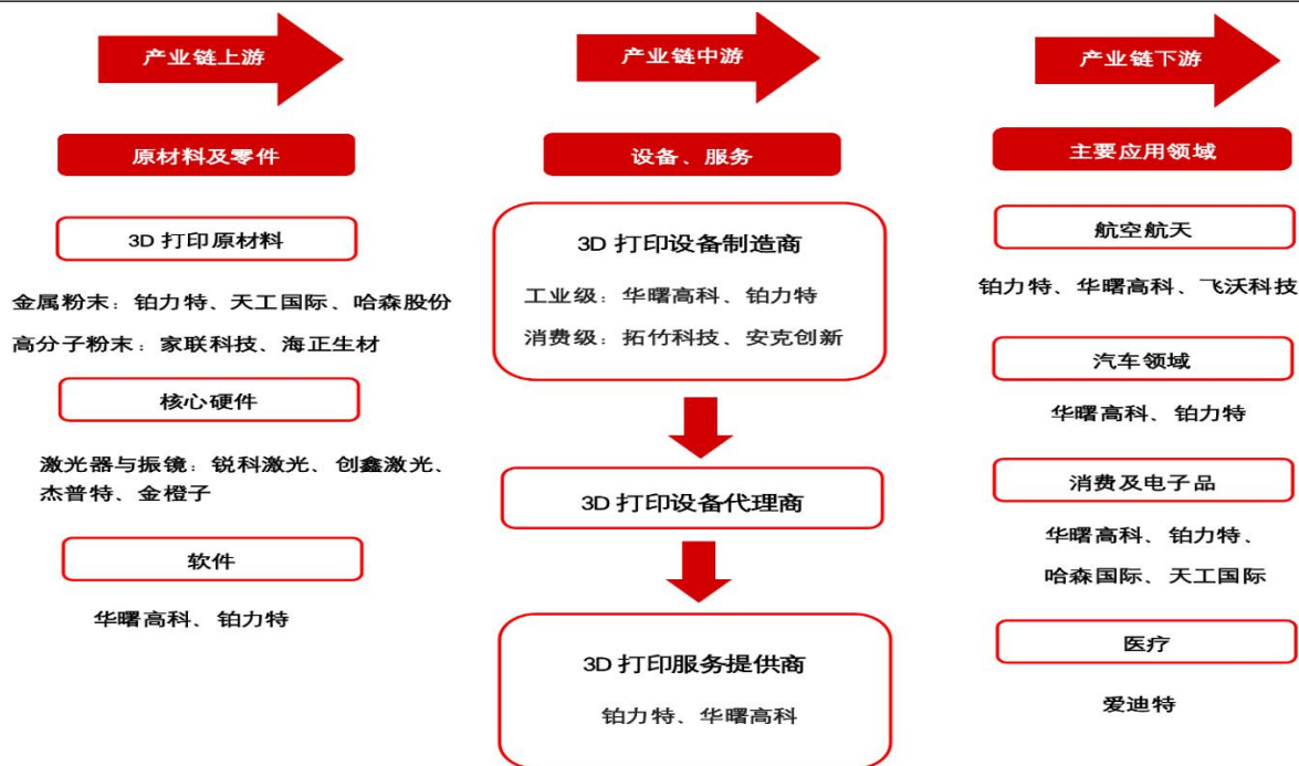
图 5：行业产业链
