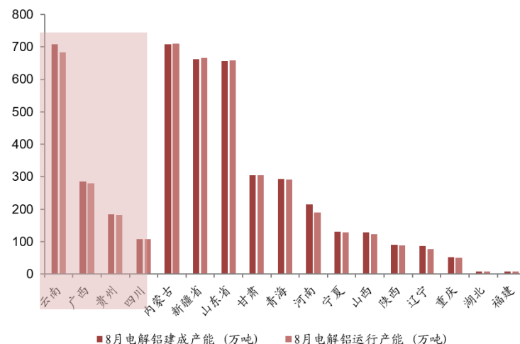
我国电解铝运行产能分布（截止至2026年8月底）
