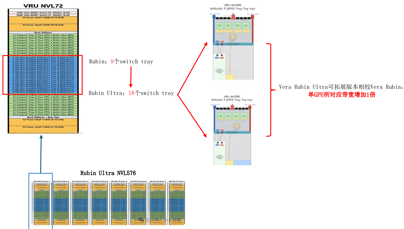
图表38：英伟达 Rubin Ultra 576 可扩展版本将增加系统带宽
