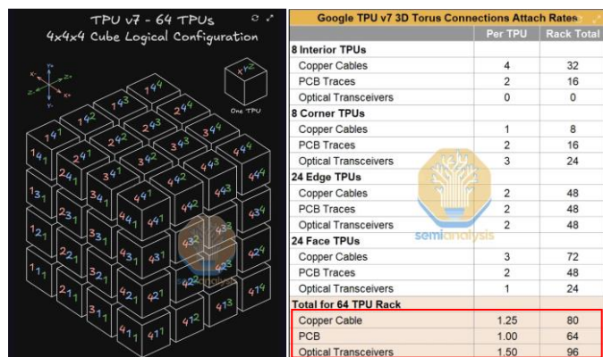
图表46：谷歌 TPU V7 采用 3D Torus 环形网络，同时采用铜缆、PCB、光模块三种物理器件
