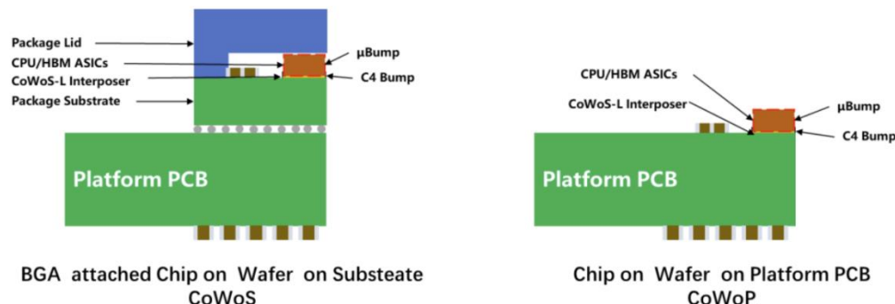
图表48：CoWoS 和 CoWoP 的对比示意图
