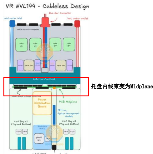
图表42：Rubin 中托盘内线束被 PCB 板取代示意图
