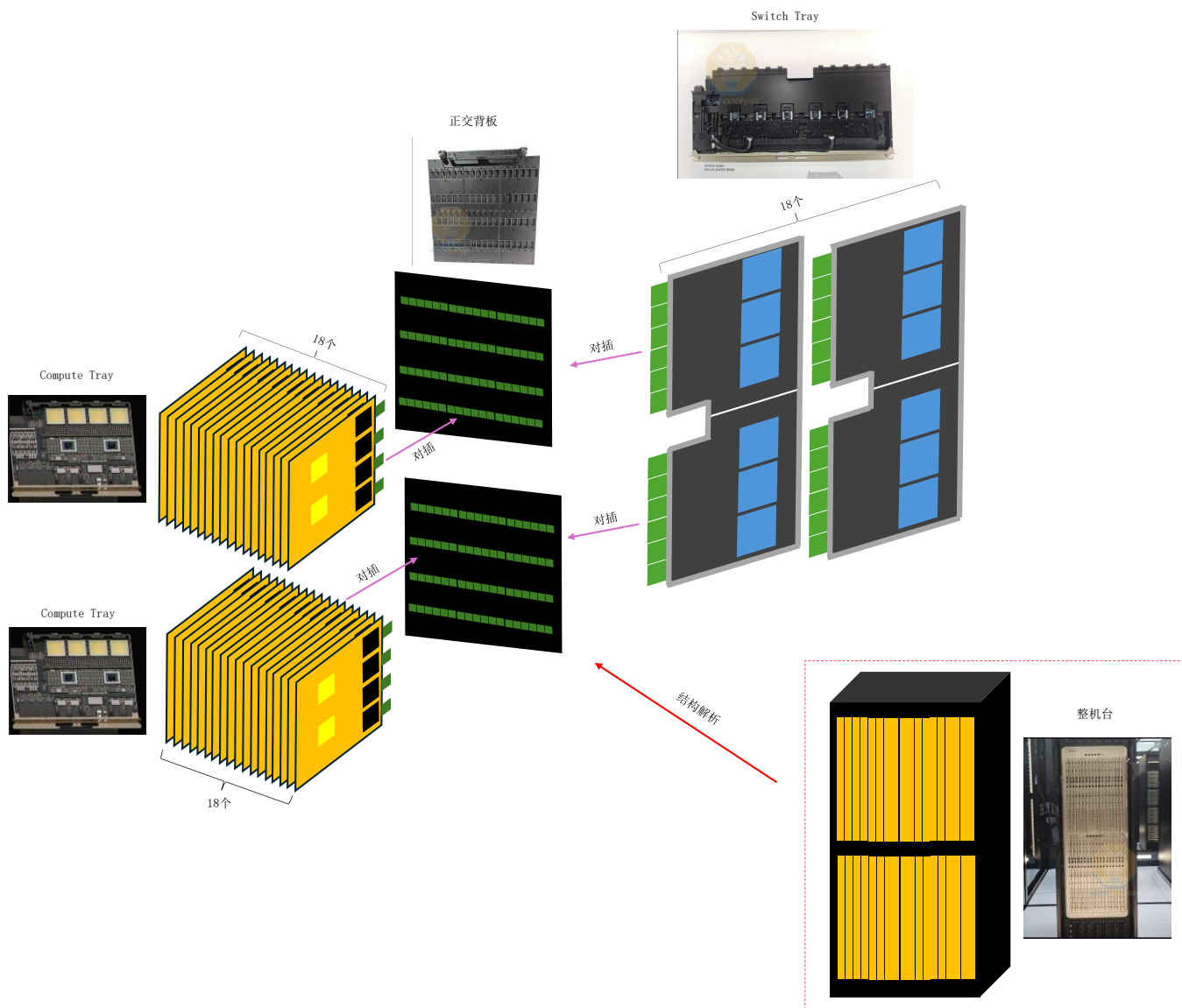
图表45: 英伟达 Kyber NVL144 核心部件结构解析
