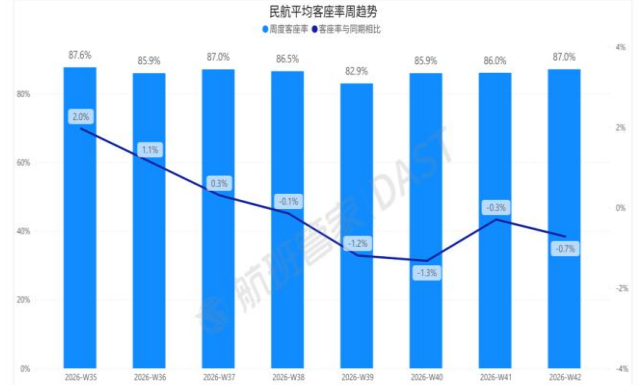
图表10: 民航平均客座率周度走势
