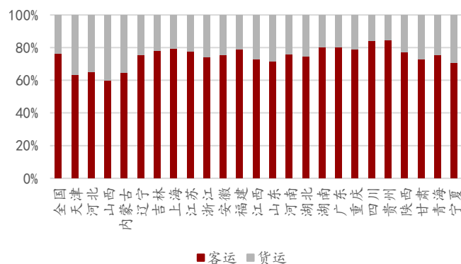
图表20:2019年我国各省市高速公路客货运车流量结构
