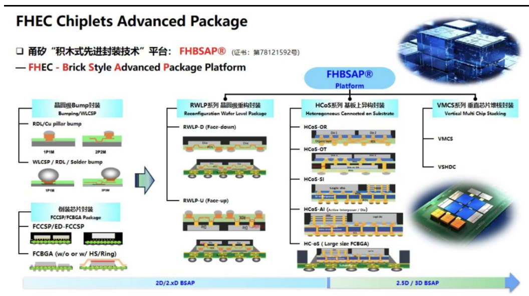
图25：基于 Chiplet 的 FHBSAP 封装平台
