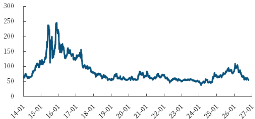
图8 国防军工（申万）指数 PE 走势图
