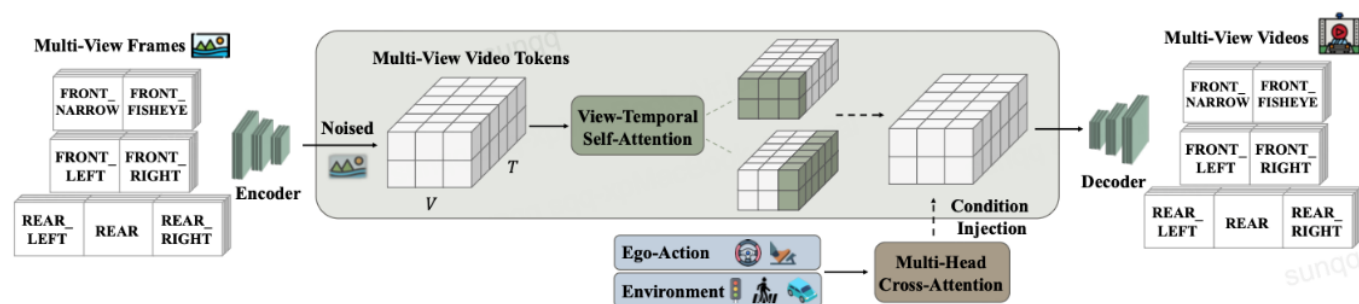
图 13：X-World 模型框架
