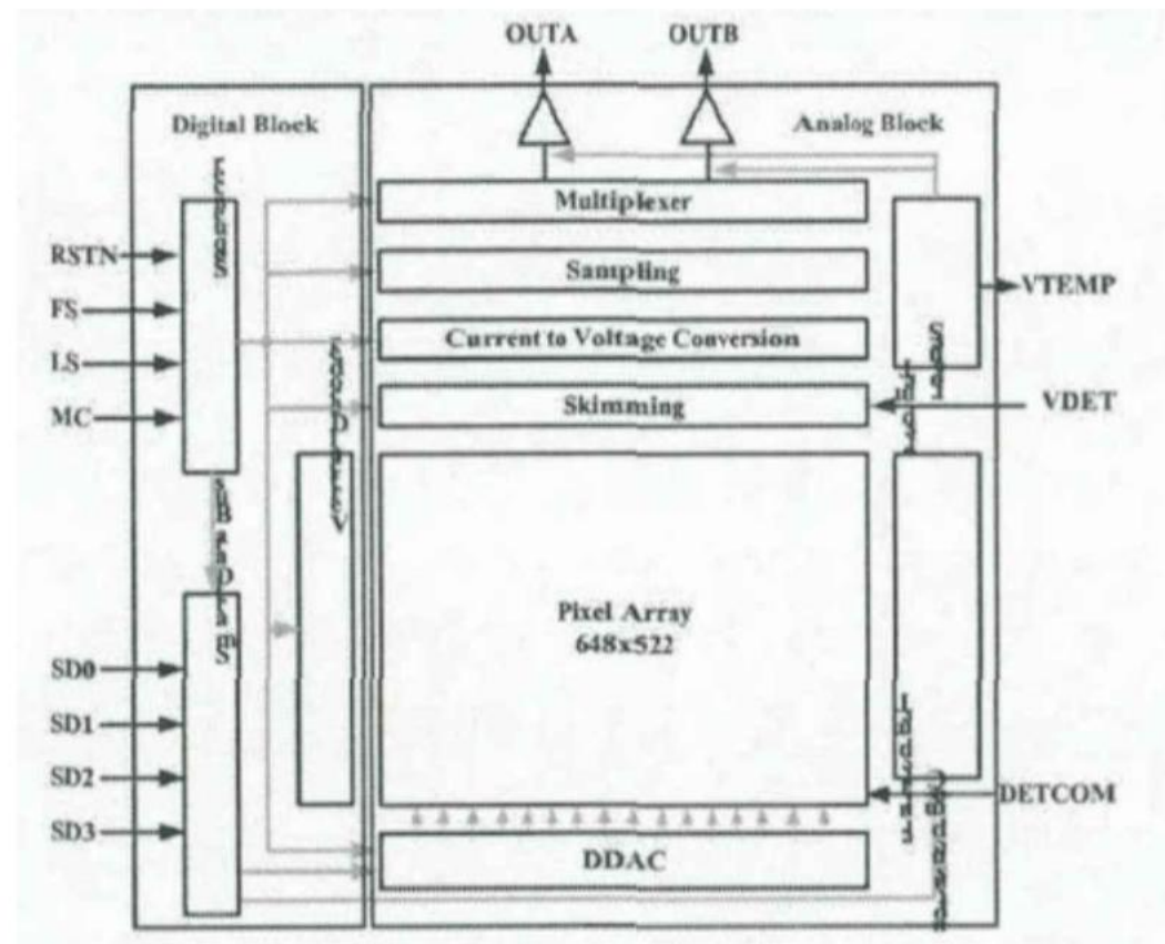
图表：读出电路架构
