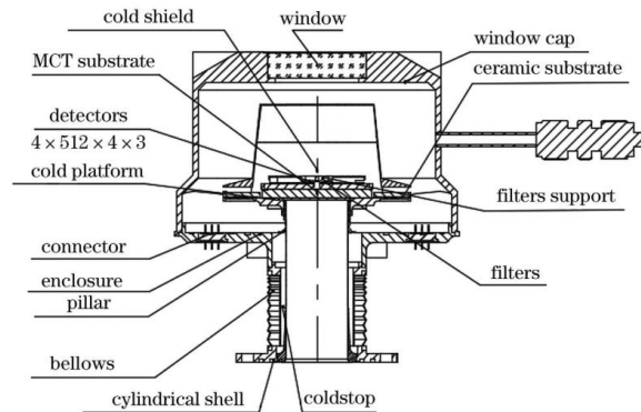
杜瓦封装结构
