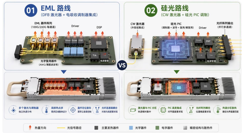
图13：EML 与硅光架构热点分布对比
