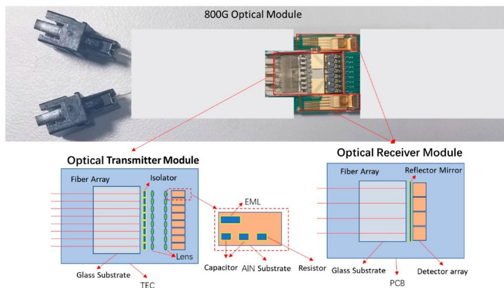
图5: EML 在光模块的位置及内部封装结构
