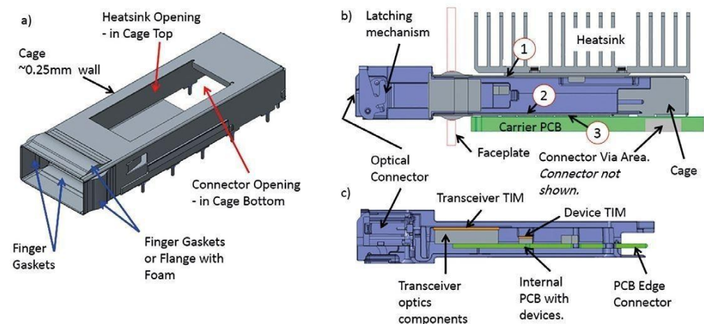
图10：光模块、Cage 与主动散热器剖面结构图
