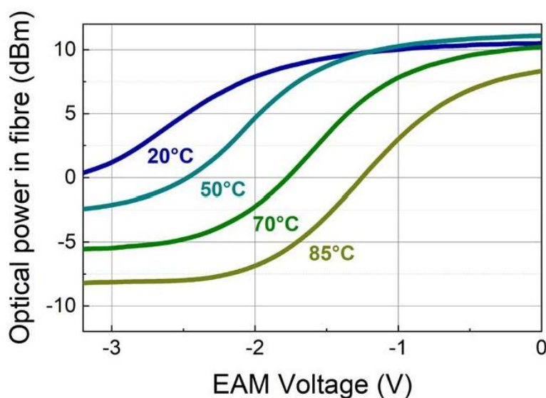
图2：不同温度下 EML 的光输出特性具有显著差异，影响性能稳定
