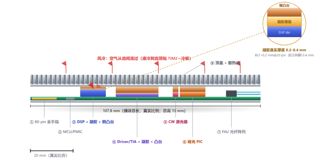
图7：光模块内部结构及散热材料应用位置
