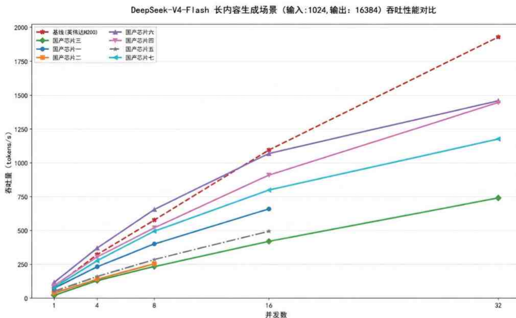
图 7 以 AISHPerf 长文档生成测试场景为例， 国产芯片吞吐率性能在中低并发场景下已接近国际主流芯片
