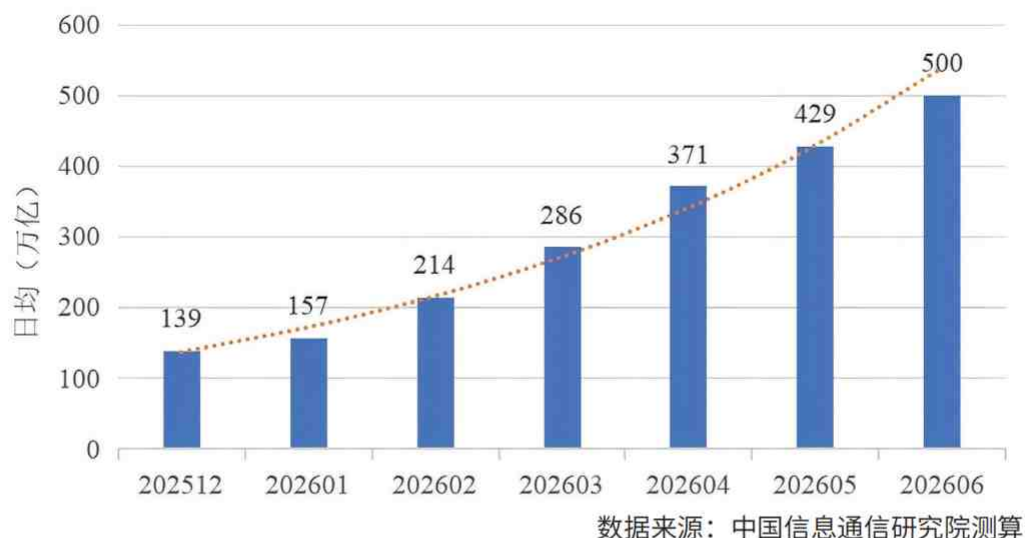
图 11 我国词元日均调用量趋势图
