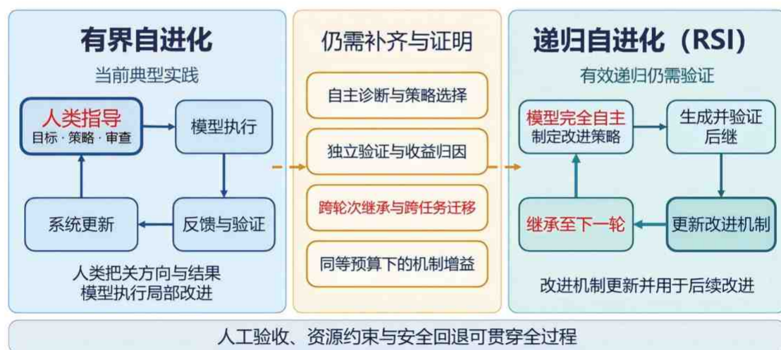
图 2 迈向递归自进化仍需可靠验证与经验继承
