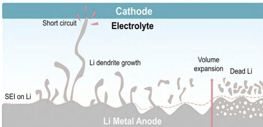
锂金属负极失效机理
