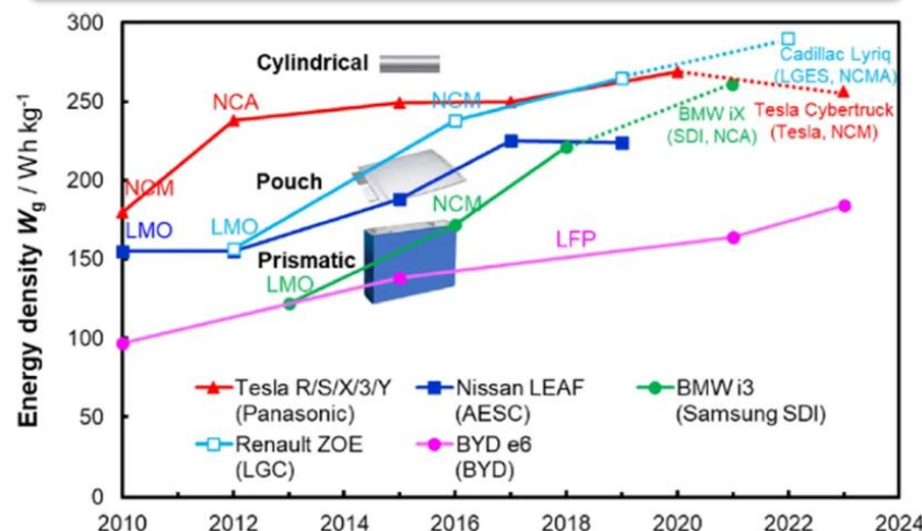
2010-2024锂离子电芯能量密度历史演进
