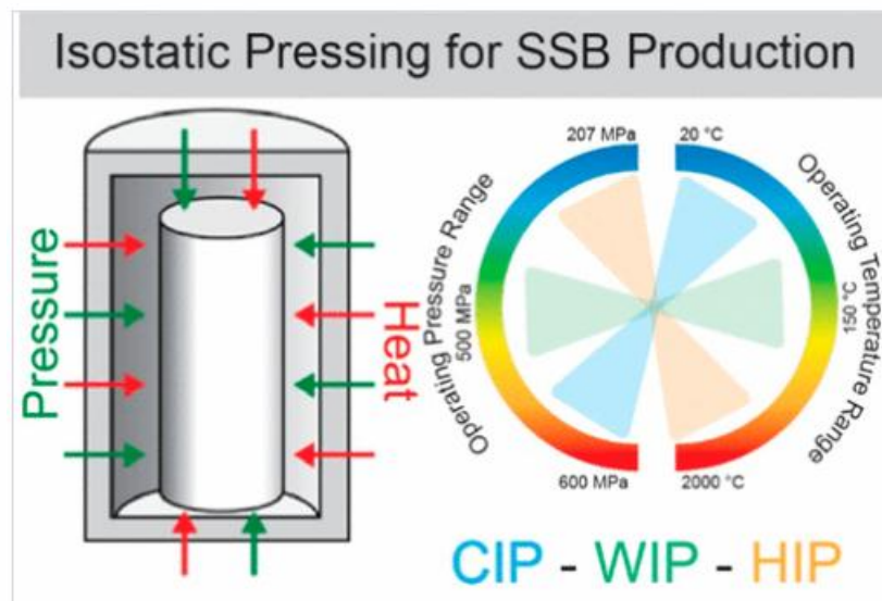
固态电池制备中等静压设备示意图
