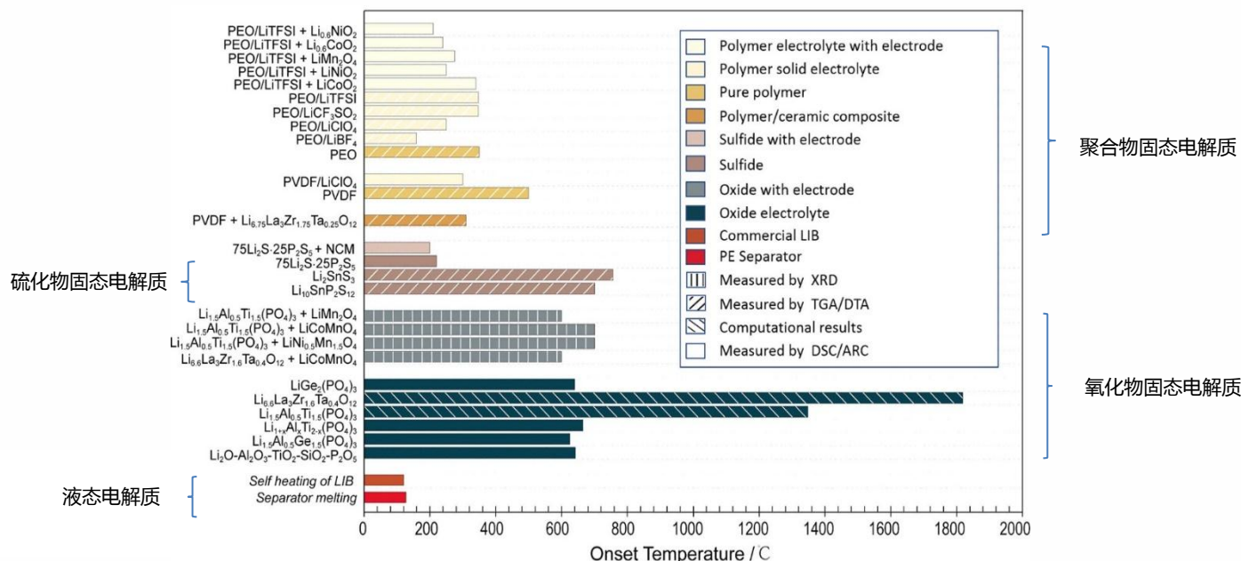
不同固态电解质（SSE）放热行为起始温度的比较
