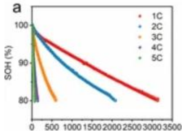
磷酸铁锂/石墨电池在1C-5C充电倍率下的性能衰减
