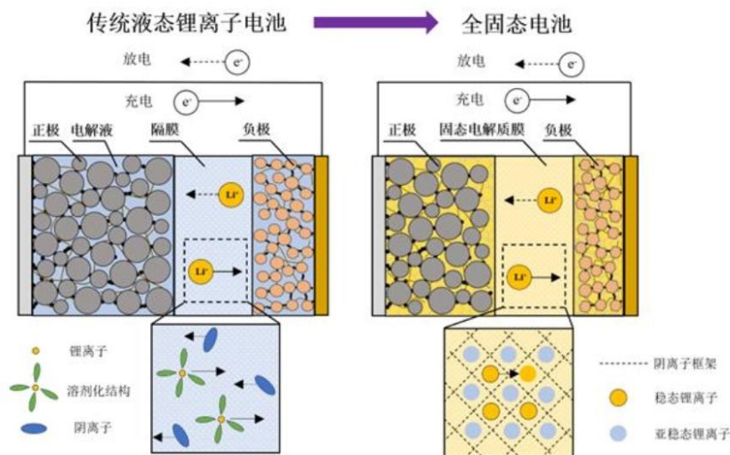
全固态锂电池结构示意图
