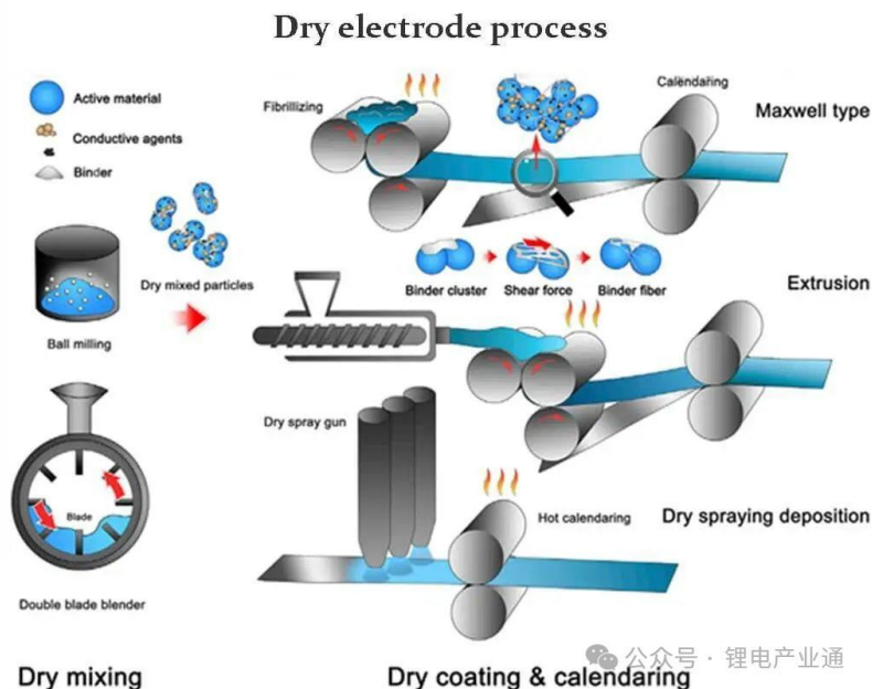
干法电极制备流程图
