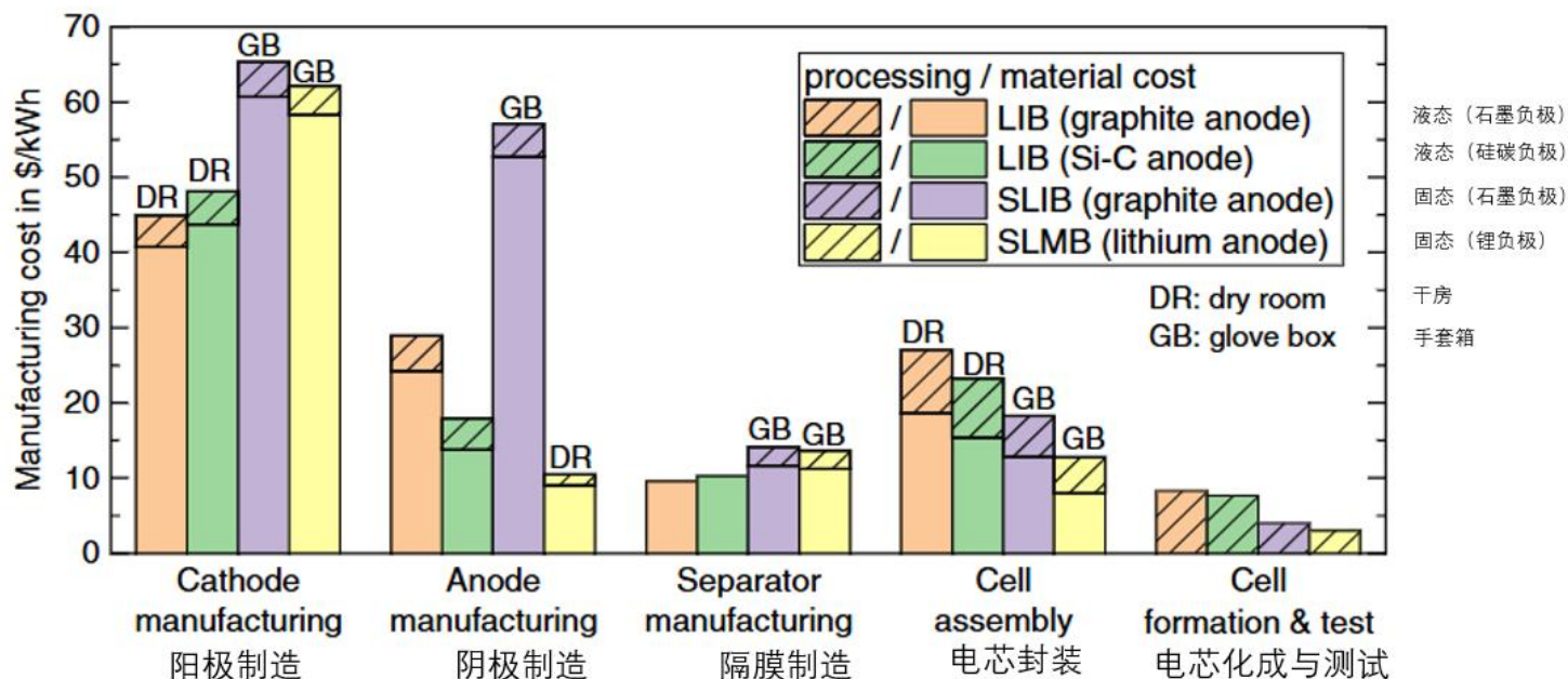
液态/固态电池成本拆分
