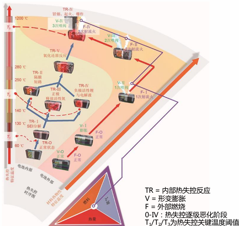
电池失效热溢时序
