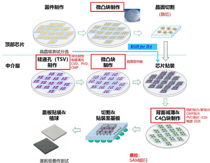
图表19：先进封装流程和新增设备需求示意图
