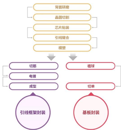
图表18：传统封装流程示意图
