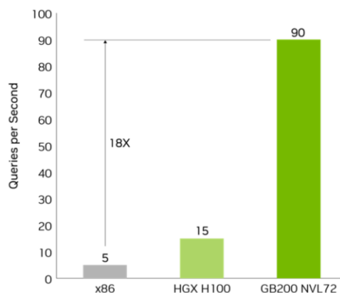
图表13: 英伟达 Blackwell B200 的查询性能显著提升
