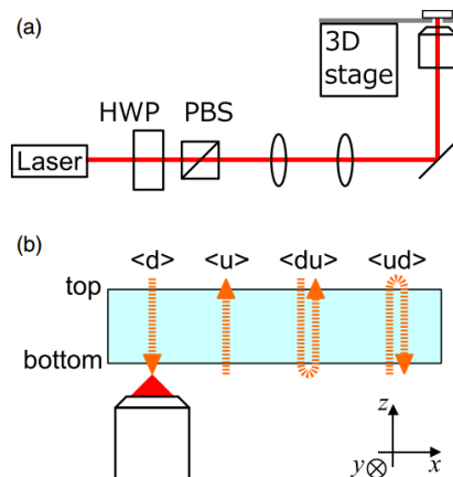
图表29：激光改性示意图
