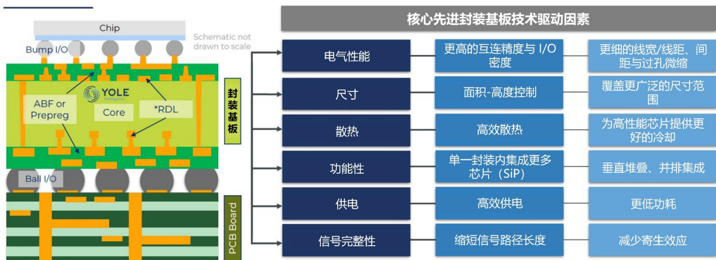
图表26：先进封装对于基板的电气性能、信号完整性等指标要求不断提升
