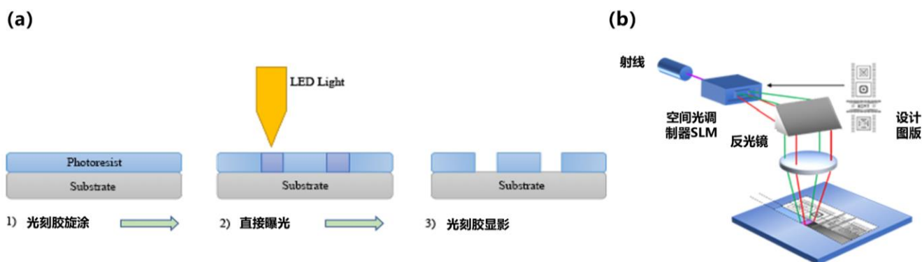
图表37：直写光刻原理示意图
