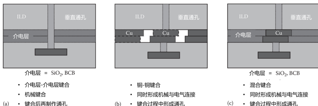
图表30：混合键合与其他两种键合方式的示意图对比
