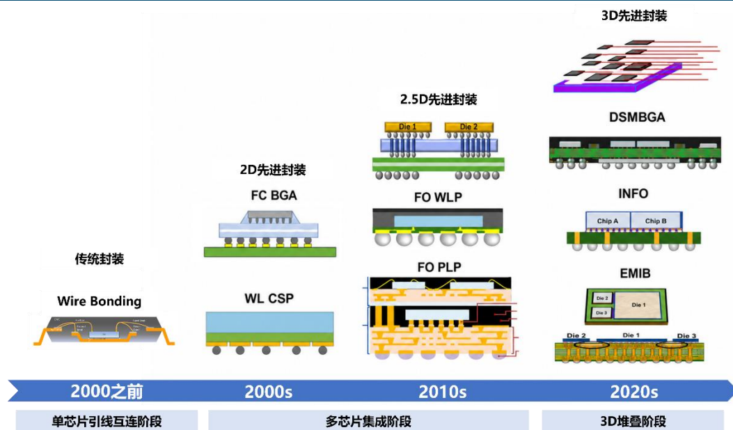
图表4：芯片级封装技术演进经历三阶段，目前已迈入 3D 堆叠阶段
