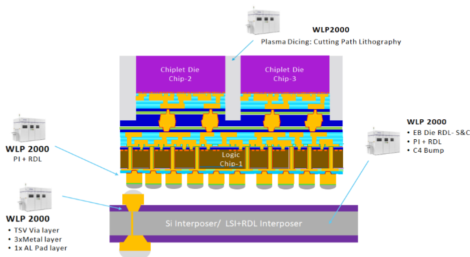
图表62：芯基微装 WLP2000 在先进封装关键制程中的应用
