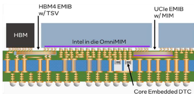
图表10：英特尔 EMIB 结构示意图
