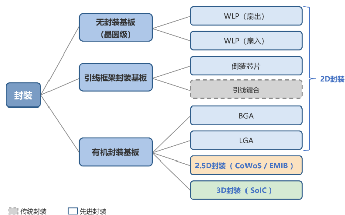
图表2：常见封装方式分类
