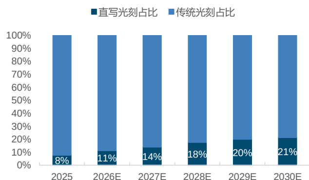
图表40：2025–2030E 全球先进封装直写光刻设备占比将不断提升
