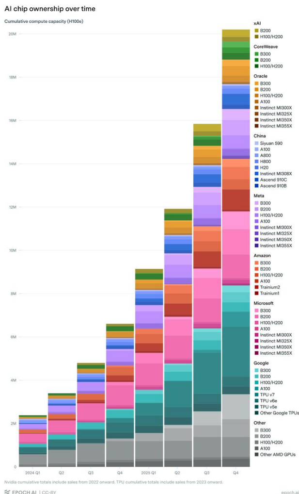
图表5: 按持有主体及芯片型号划分的AI 累计算力 (H100 等效)
