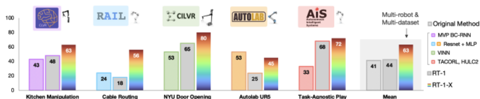
图表11: Google RT-1 与 RT-1-X 在小数据集场景下的成功率对比
