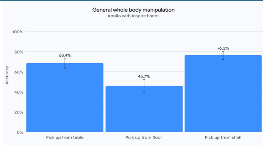
图表13: Robotics 2 搭载 Inspire 灵巧手的全身操作任务成功率
