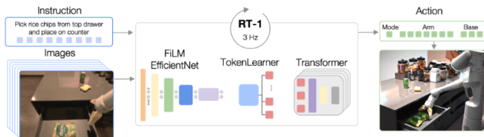
图表8: Google RT-1 架构
