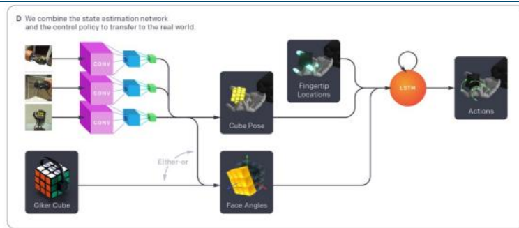
图表7: OpenAI 结合视觉状态估计与控制策略将机械手迁移至真机
