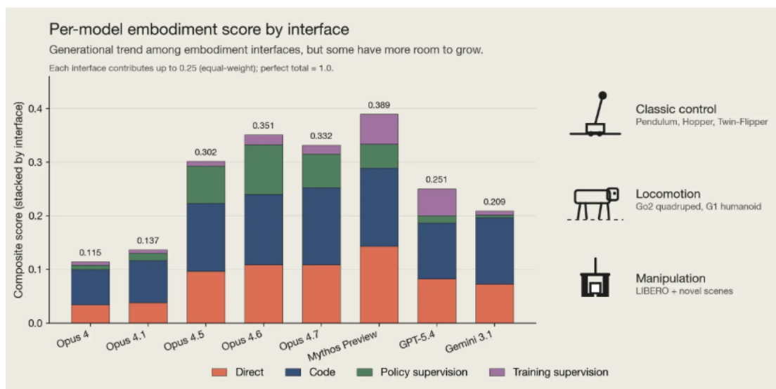
图表15: Anthropic Embody 测评各大模型机器人控制能力
