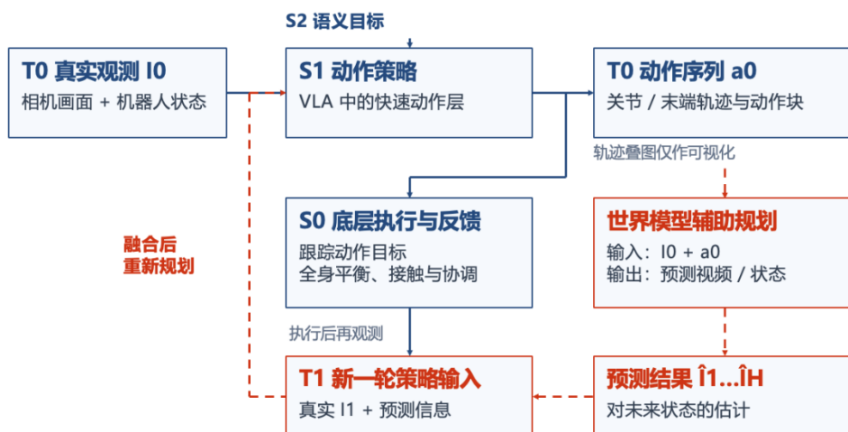
图表25: Helix S0-S2 架构
