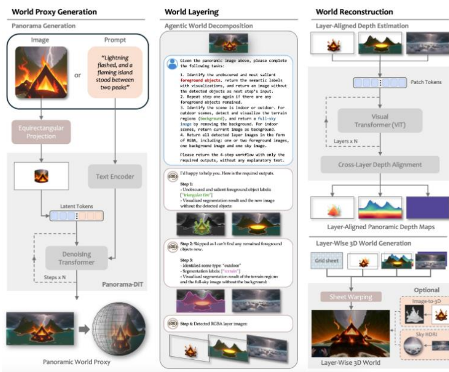
图表3: HunyuanWorld1.0 架构
