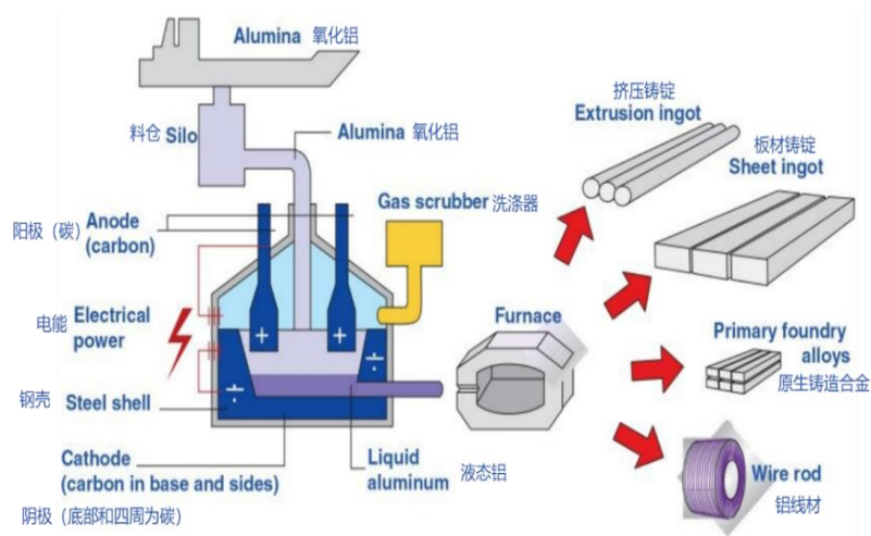
图 1：铝工艺生产流程图
