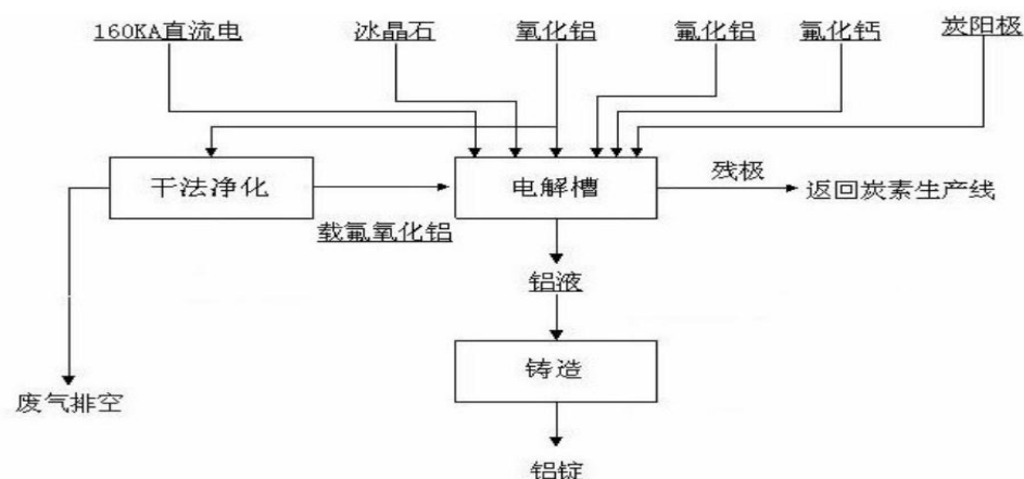
图 3：霍尔-埃鲁法电解铝工艺图
