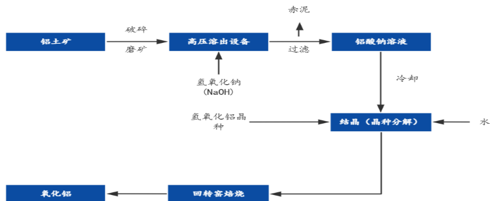
图 2：拜耳法生产氧化铝
